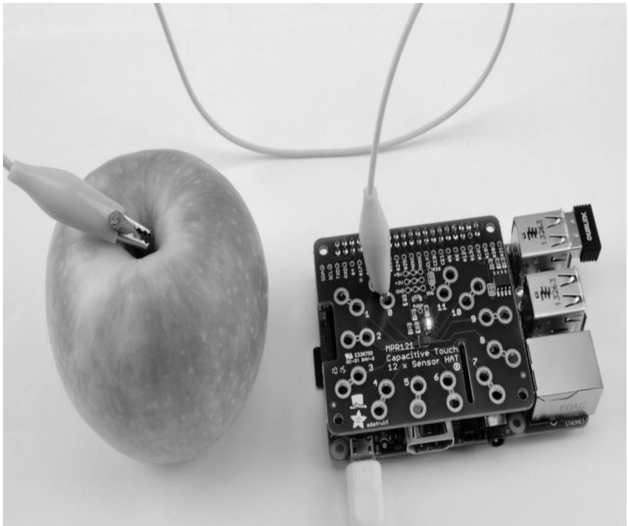
图13-25 连接到苹果上面的Adafruit Capacitive Touch HAT
