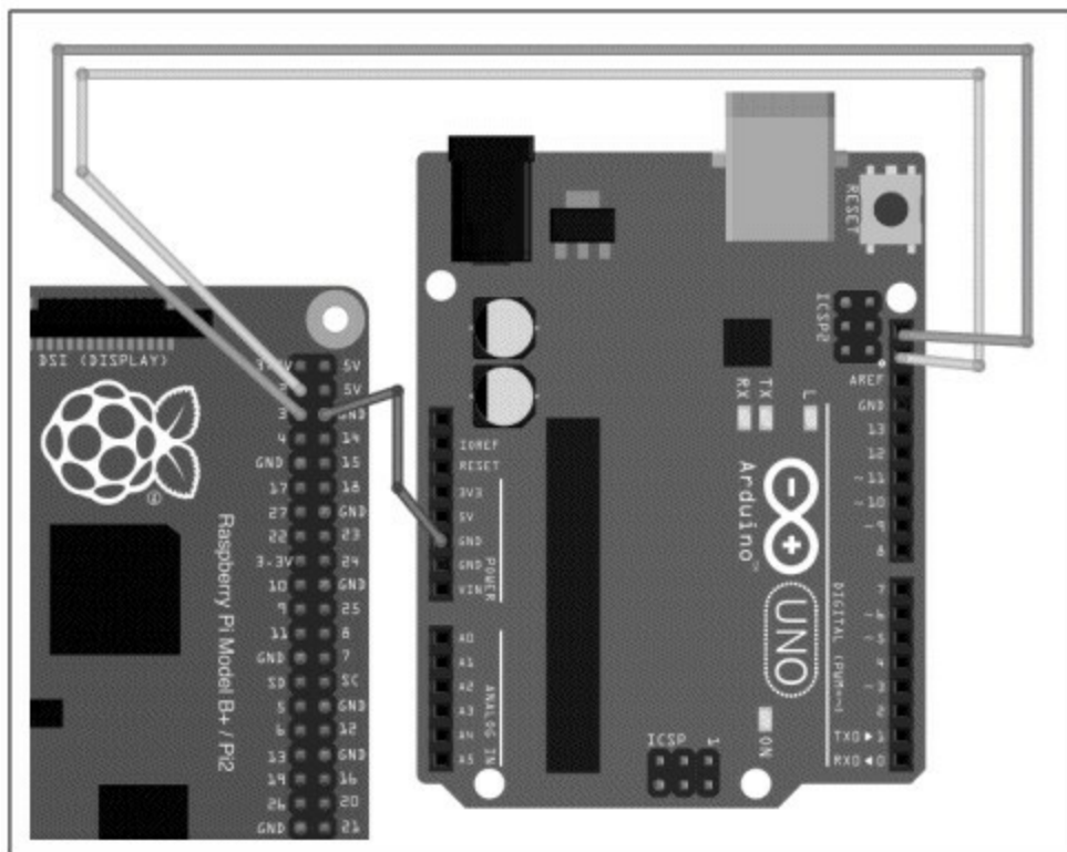
图16-16 Arduino I2C通信布线图
