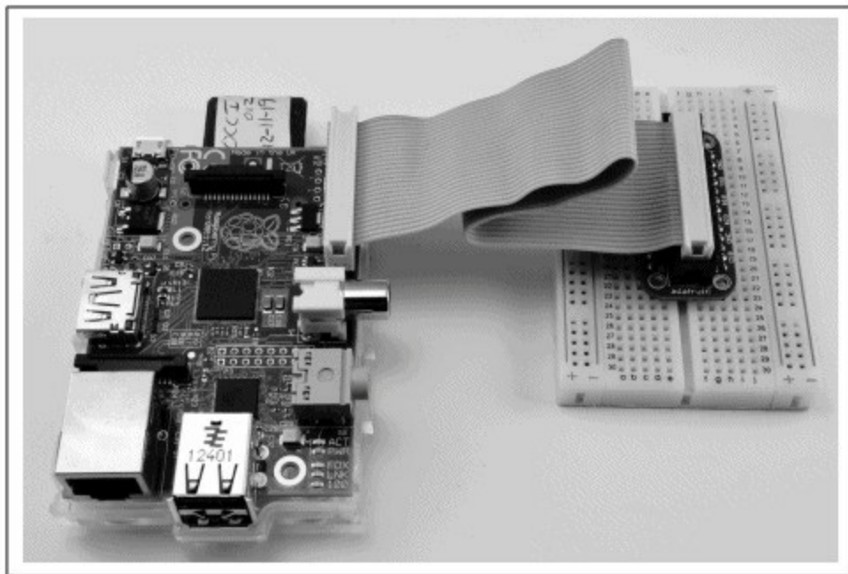
图9-10 利用排线连接树莓派和面包板
