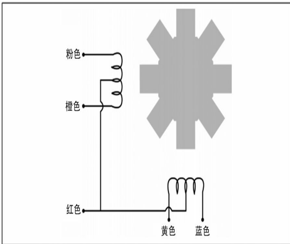
图11-13 步进电机
