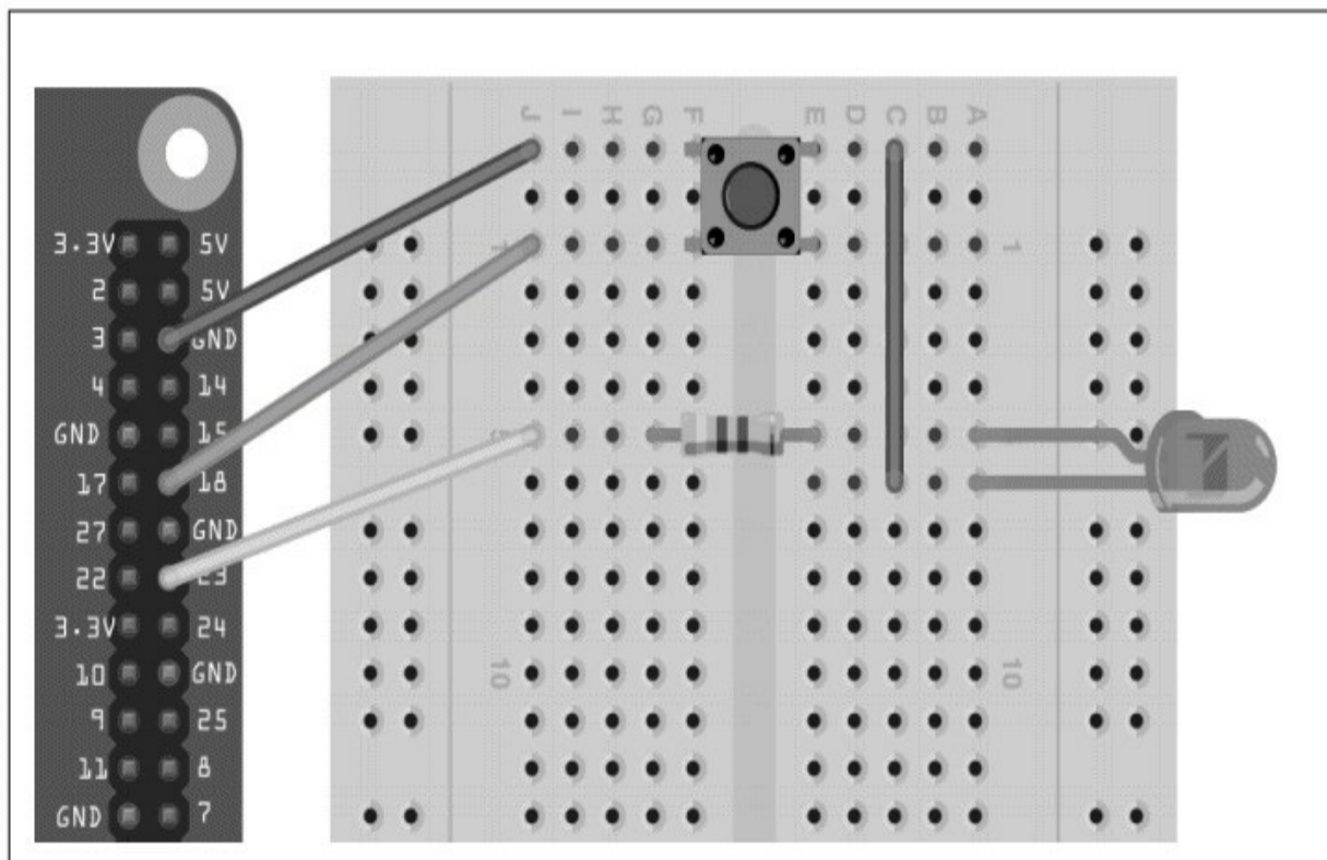
图12-4 将按钮开关和LED连接至树莓派
