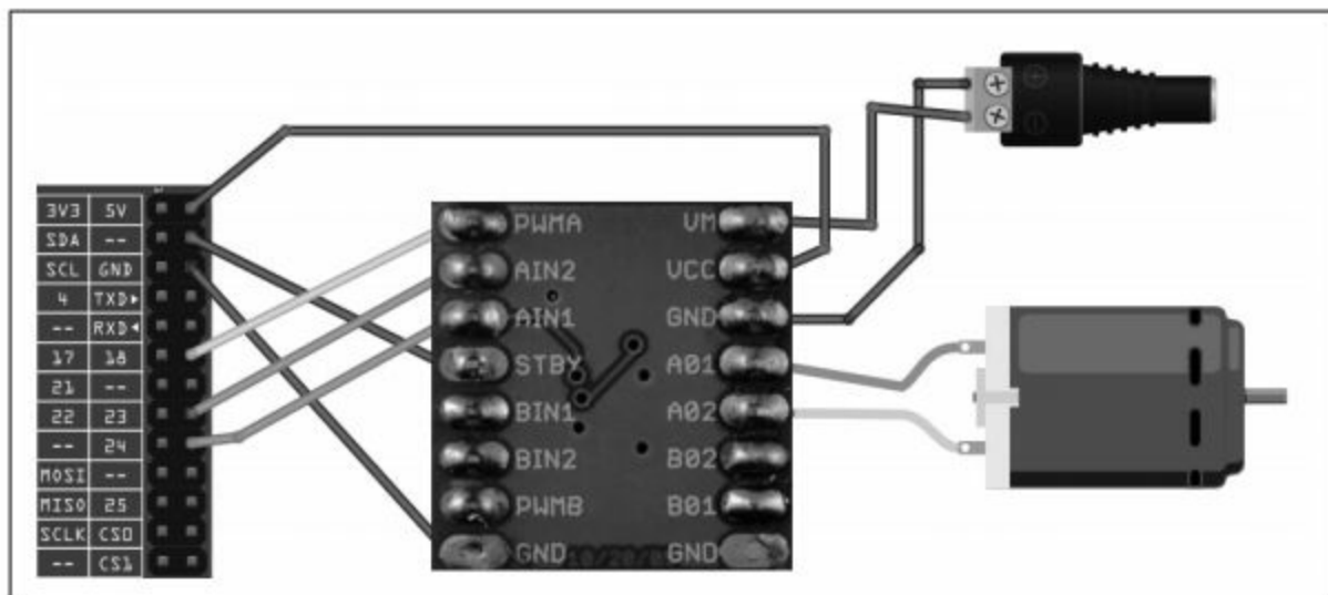
图11-9 连接SparkFun电机控制器
