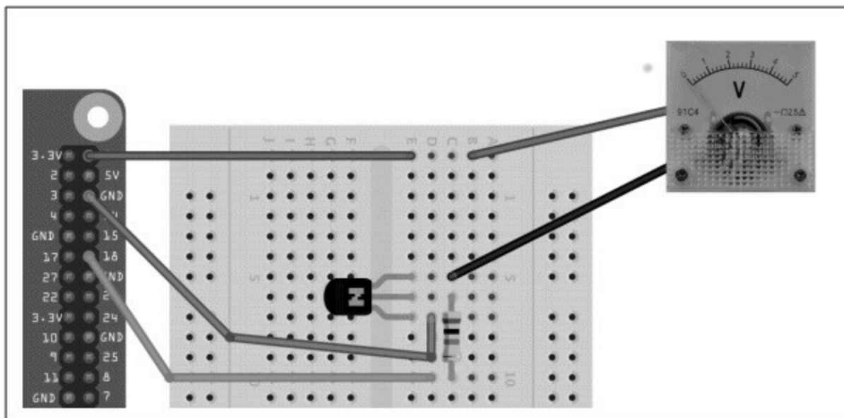
图10-15 在3.3V GPIO上使用5V电压表
