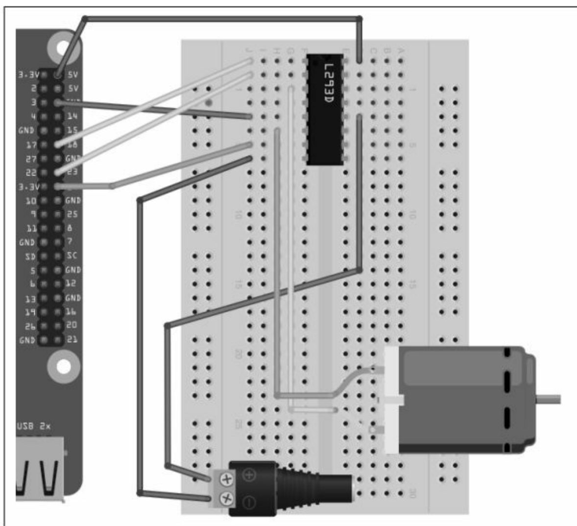
图11-8 使用L293D芯片控制电机
