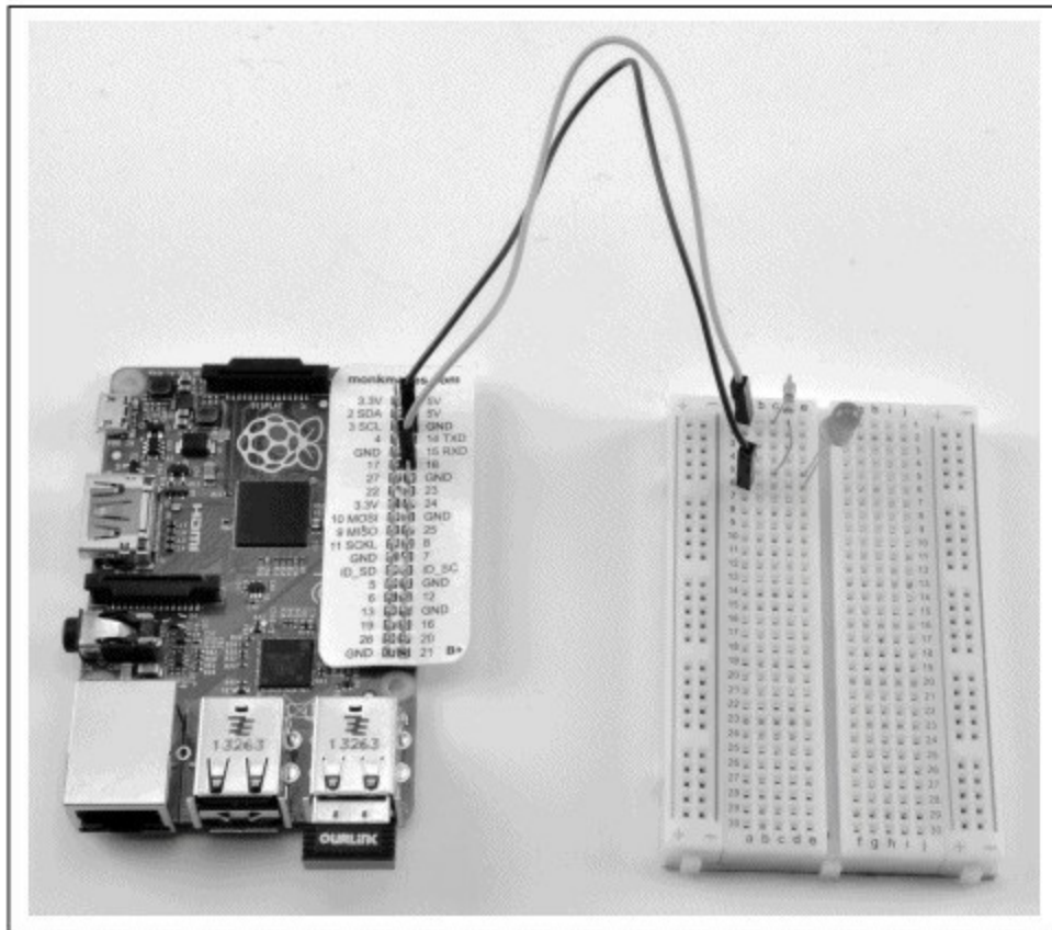
图9-9 使用male-to-female跳线连接树莓派和面包板
