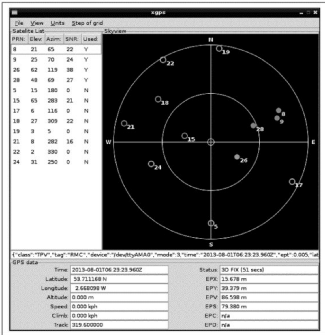
图12-17 利用xgps浏览GPS数据
