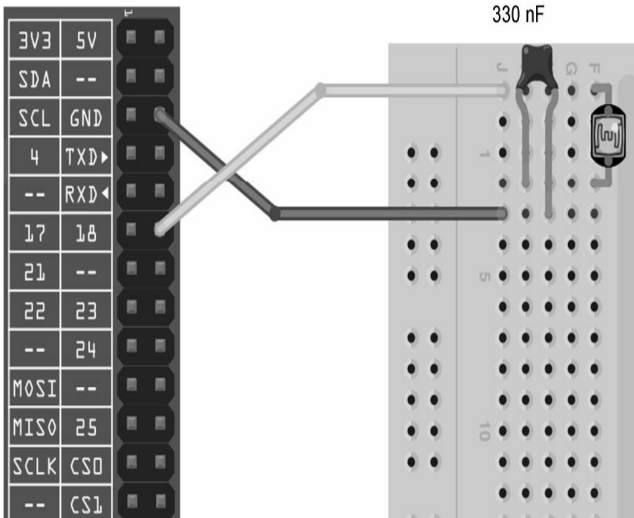
图13-5 简化后的光传感器
