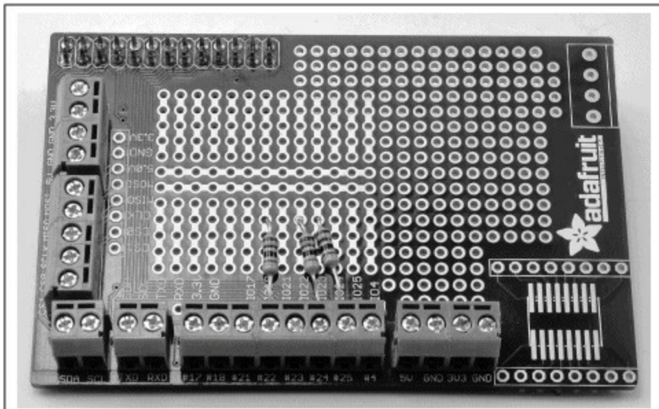
图9-25 已焊接到Pi Plate上面的电阻
