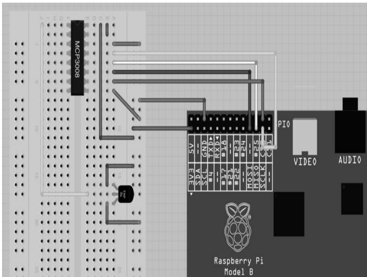
图13-15 使用TMP36与ADC
