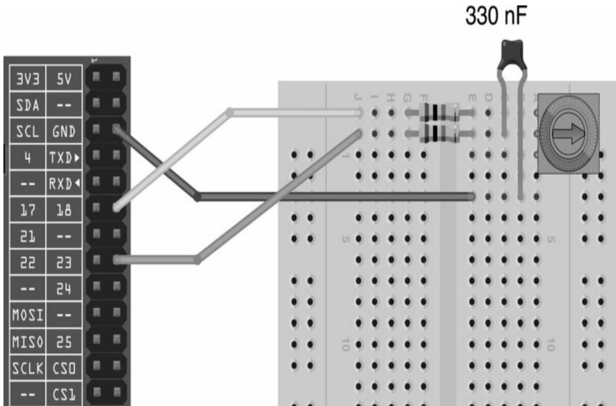
图13-1 在树莓派上测量阻值
