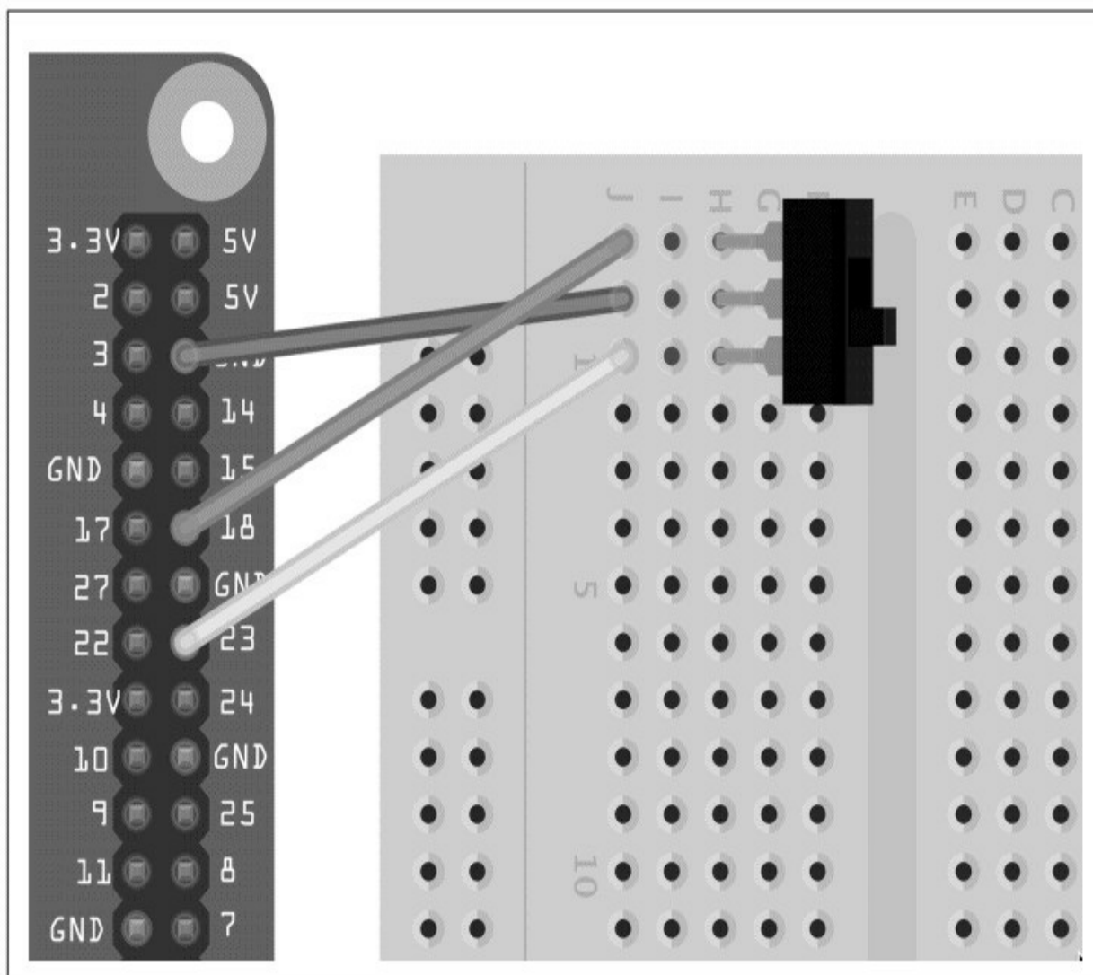
图12-6 连接三位开关到树莓派
