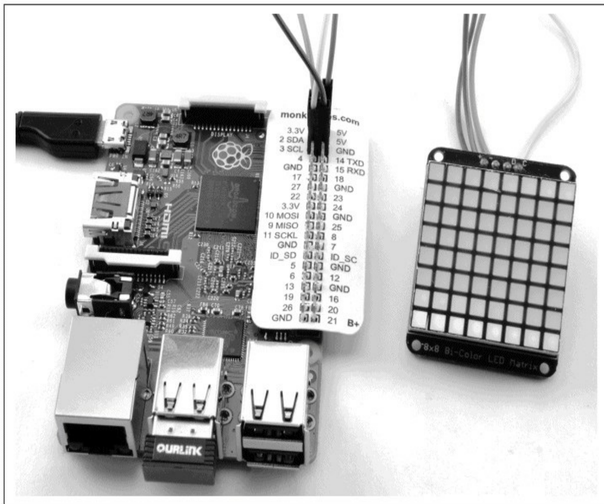
图14-2 连接树莓派的LED矩阵显示设备
