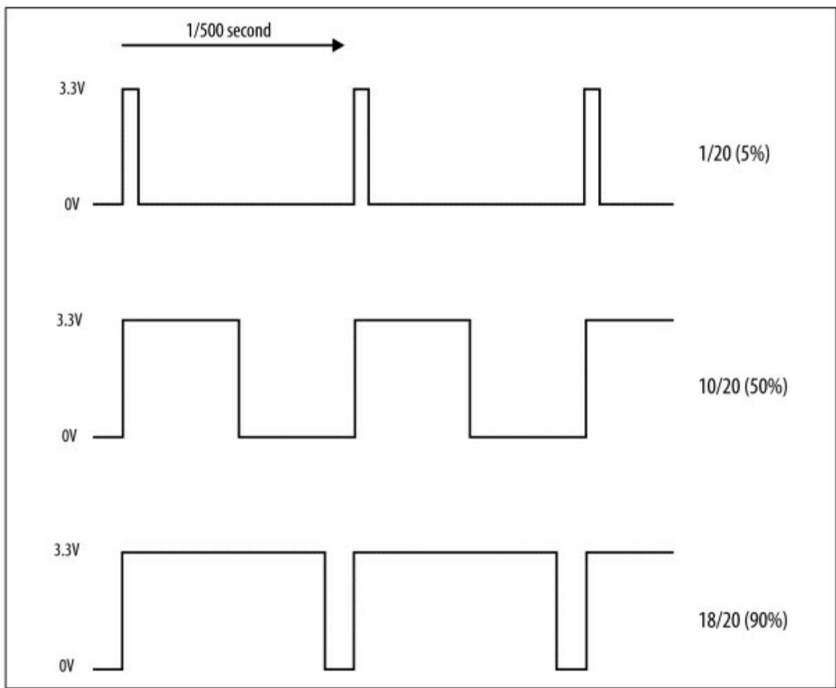
图10-2 脉冲宽度调制
