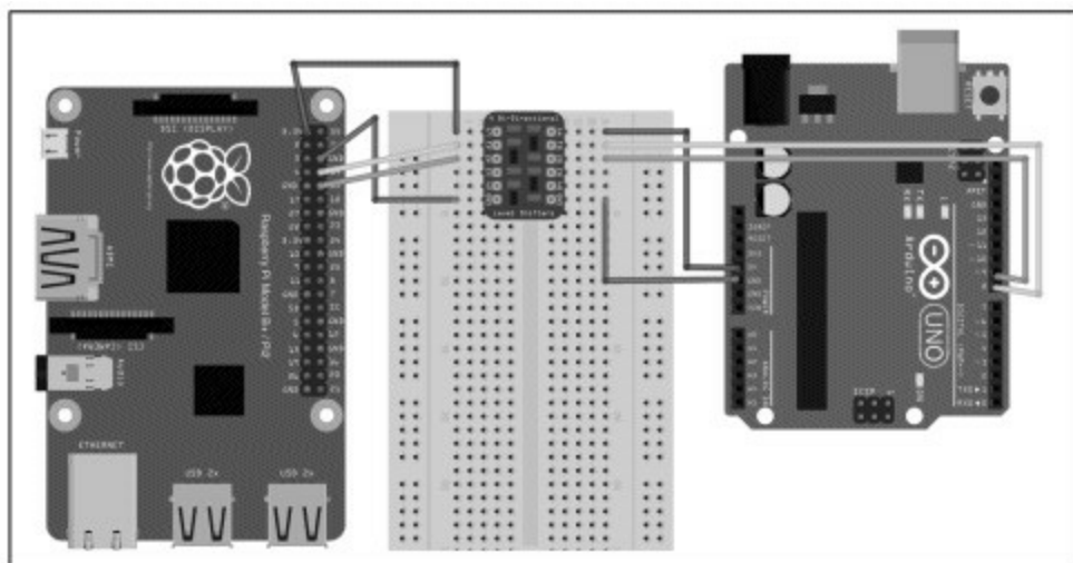
图16-7 利用电平转换模块与Arduino进行串行通信的布线图
