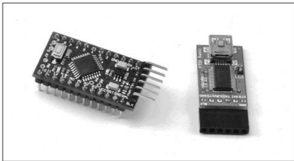
图16-17 Arduino Pro Mini与编程接口
