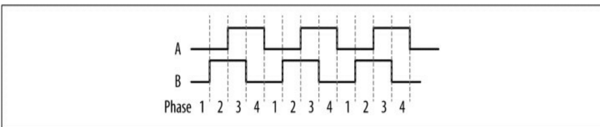
图12-11 正交编码器工作原理
