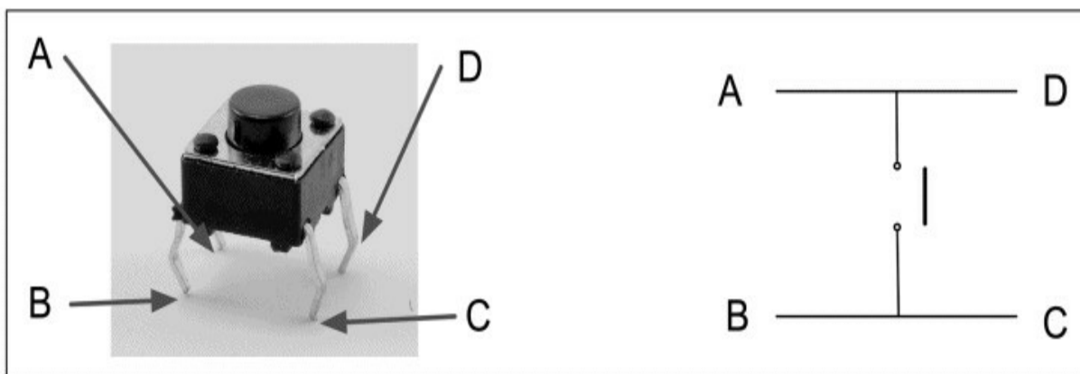
图12-3 轻触按钮开关
