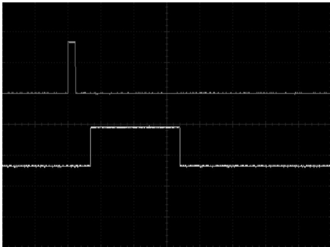
图13-24 触发和回波的示波器跟踪图
