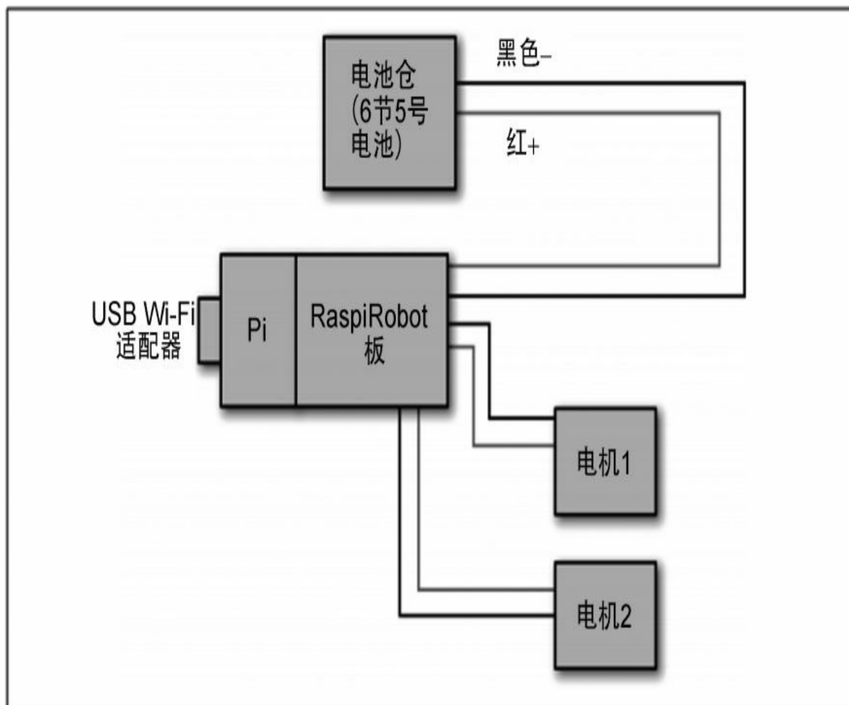
图11-17 机器人小车布线图
