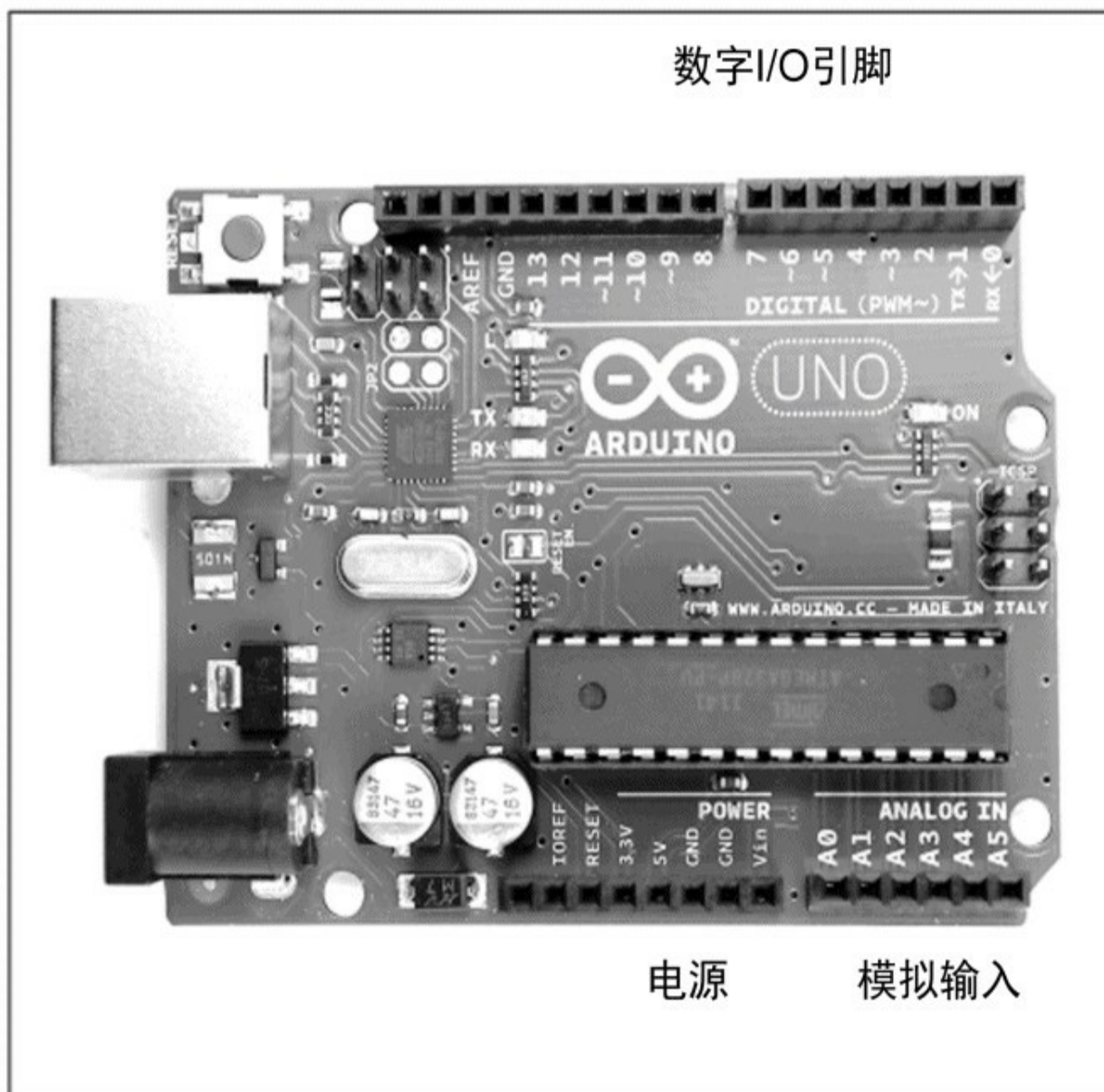
图16-4 Arduino Uno上的I/O引脚
