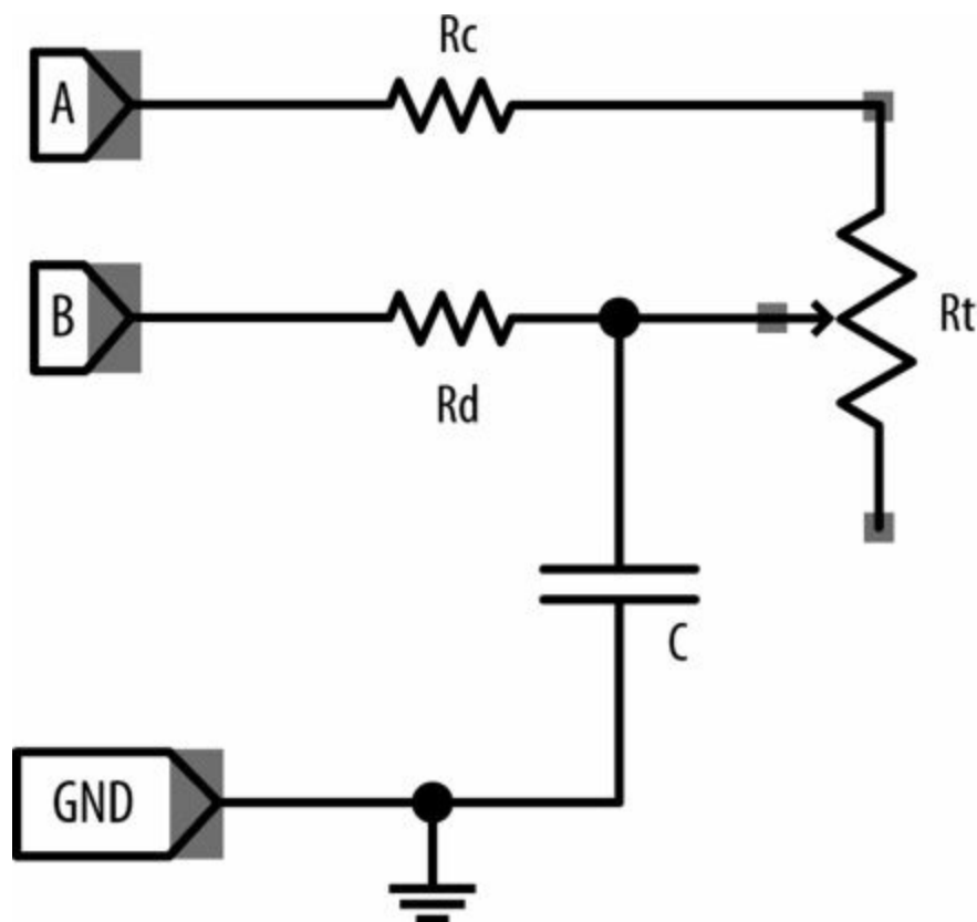
图13-2 利用阶跃响应测量电阻
