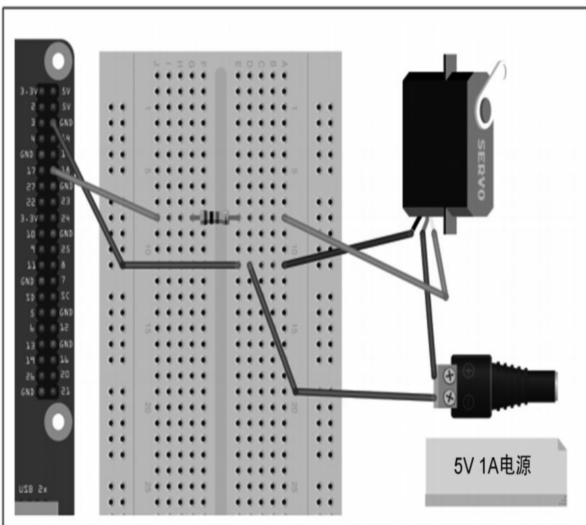
图11-2 控制伺服电机
