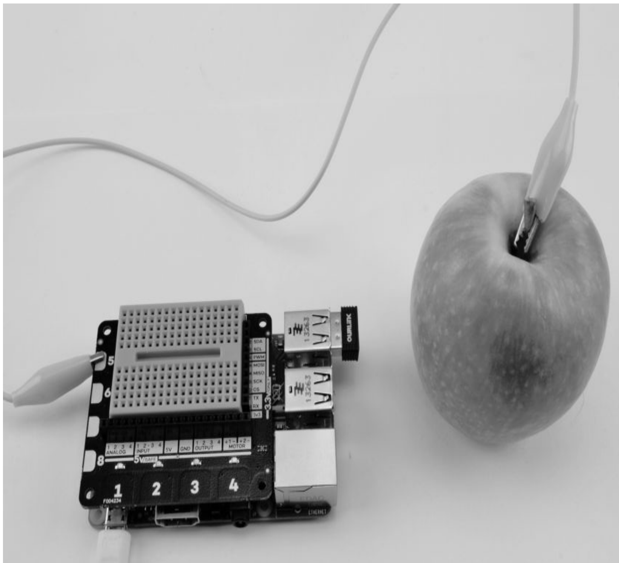
图13-26 连接水果的Explorer HAT Pro
