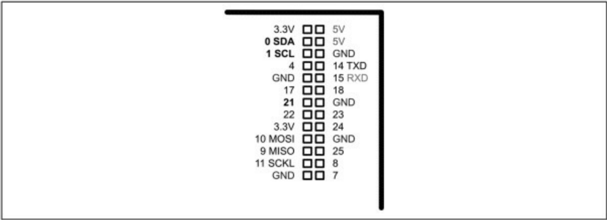
图B-3 B型树莓派第一版的GPIO引脚
