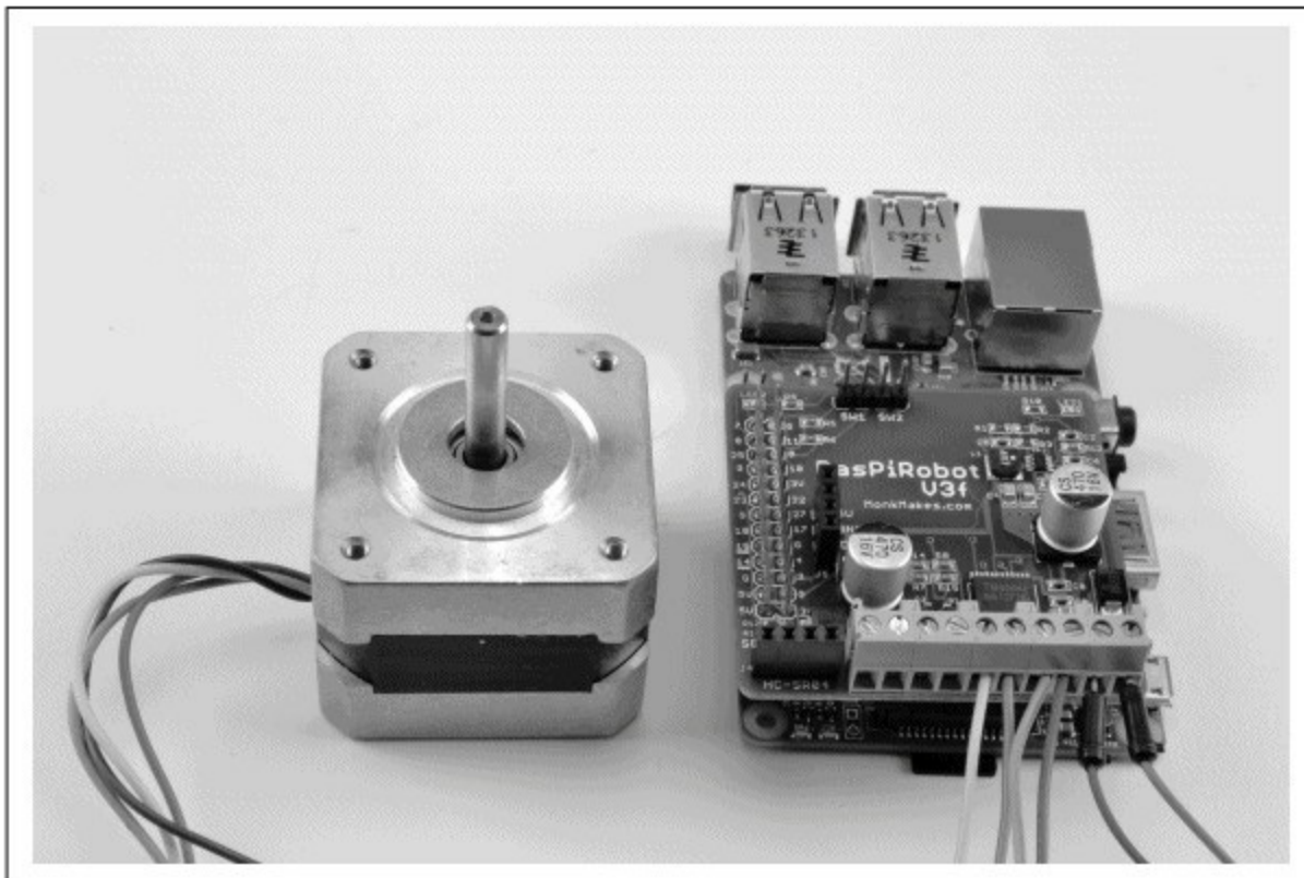
图11-16 使用RaspiRobot板控制双极步进电机
