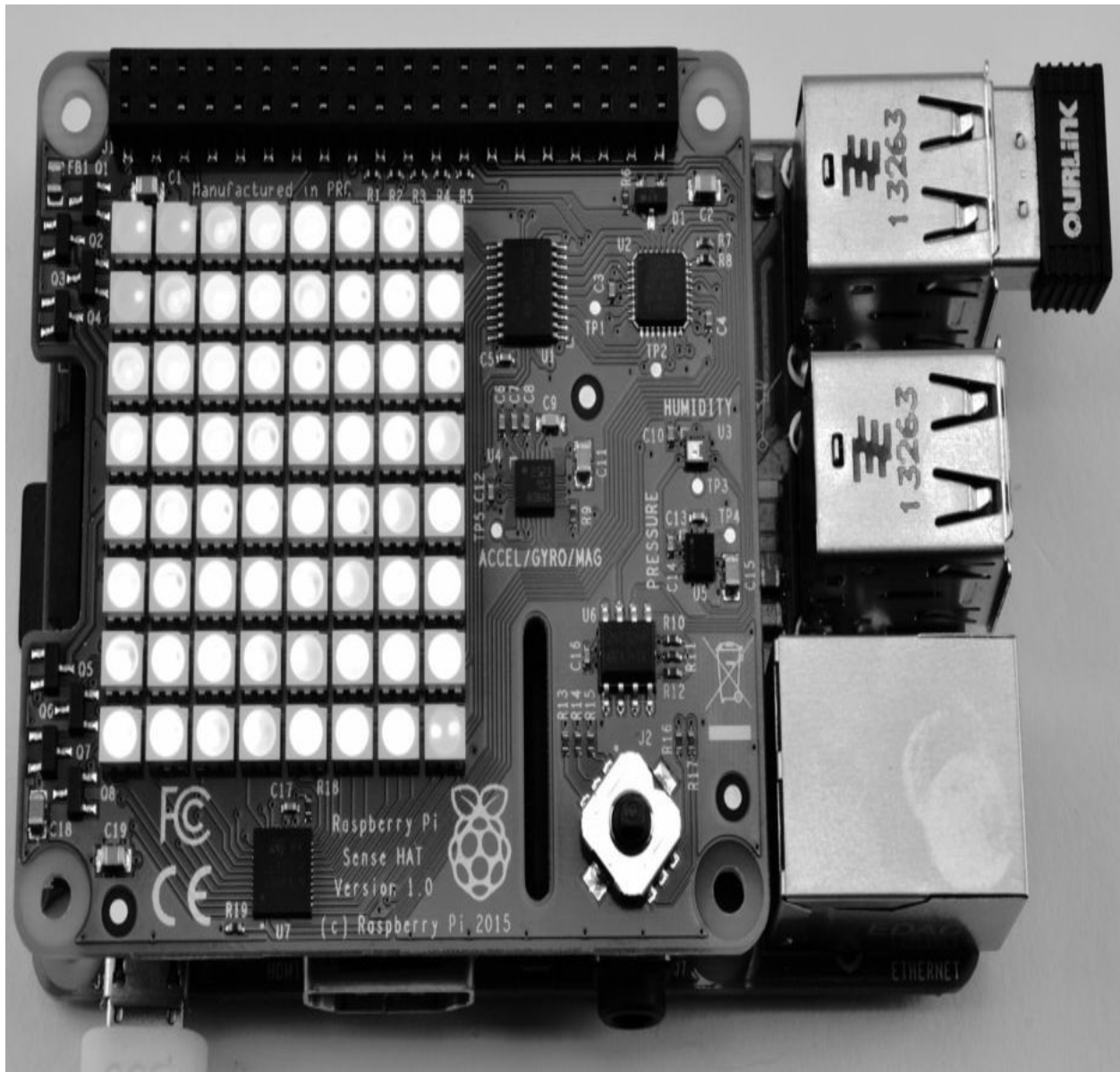
图13-16 Sense HAT
