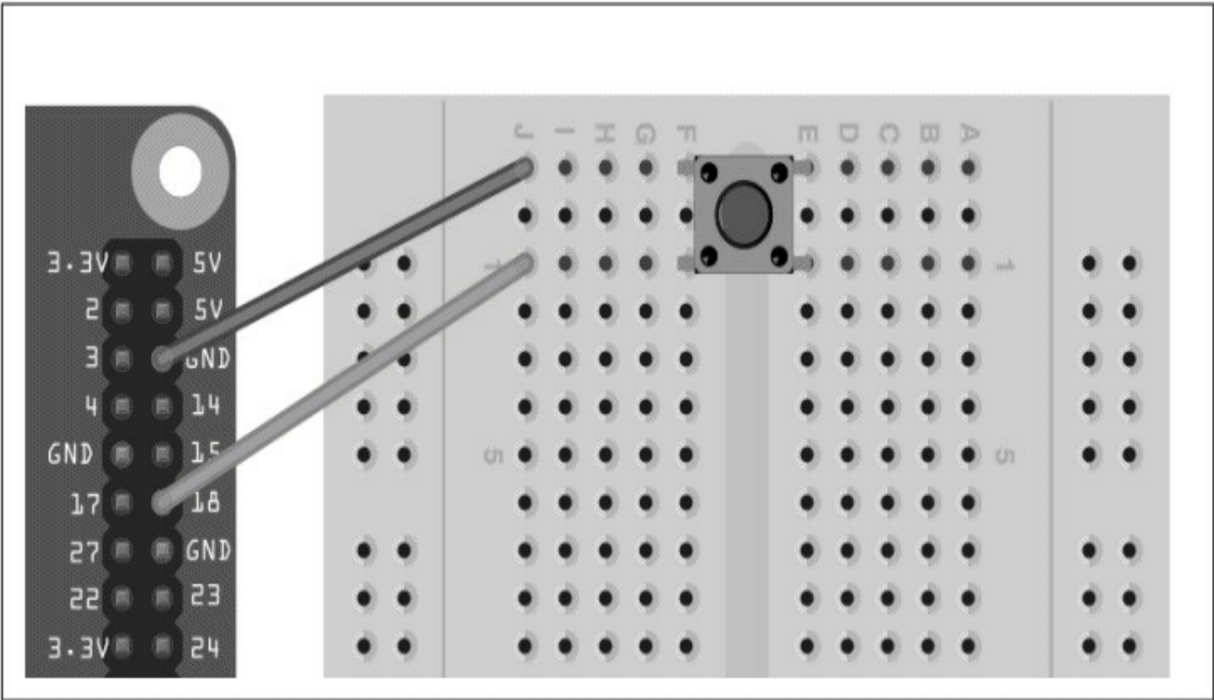
图12-1 为树莓派连接按钮开关
