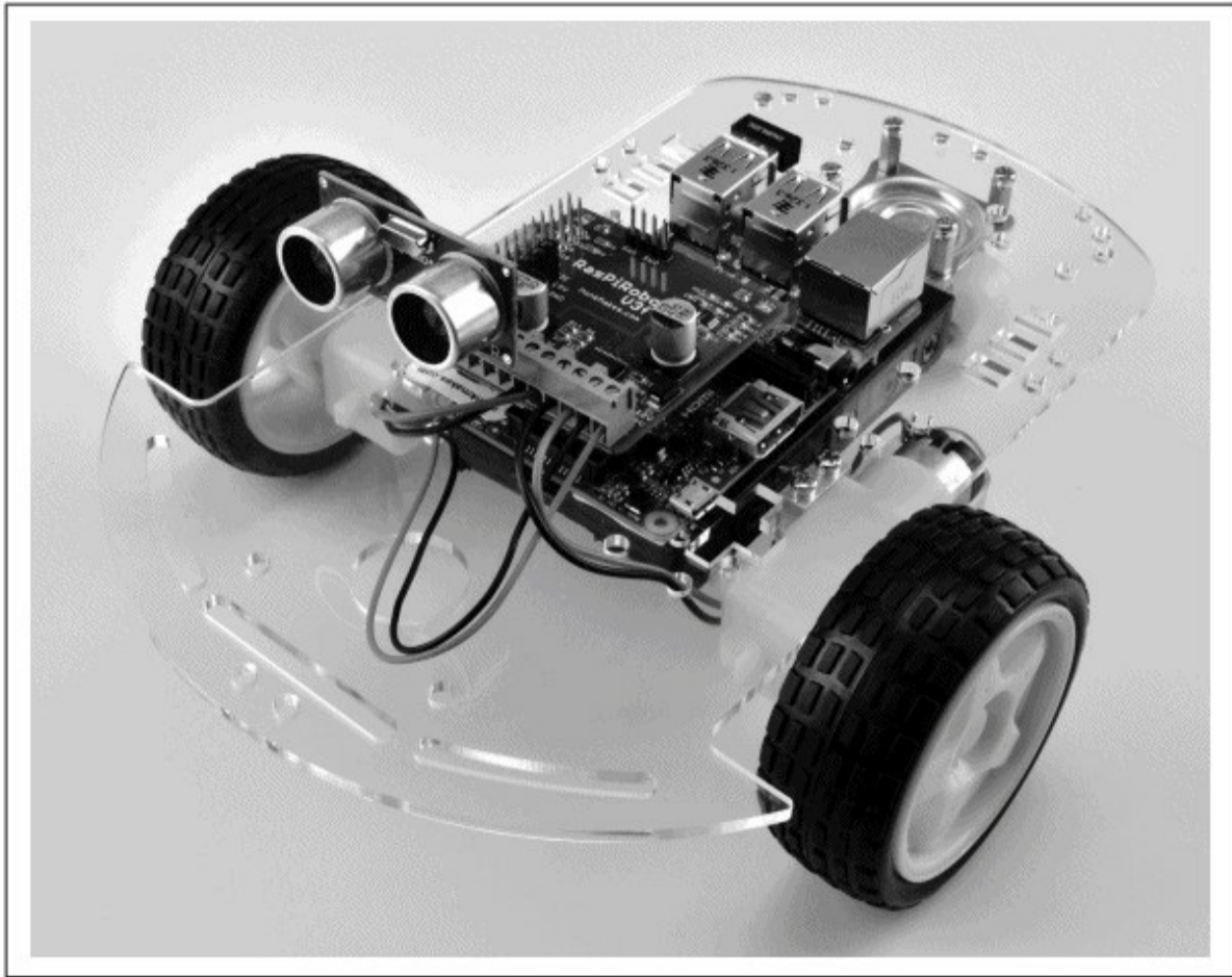
图11-18 完成后的机器人
