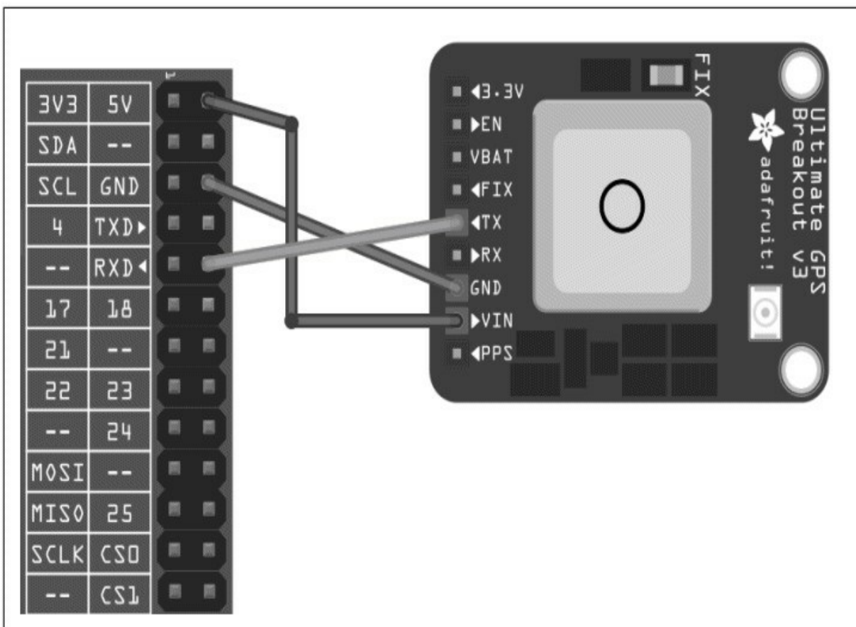
图12-15 将GPS连接至树莓派
