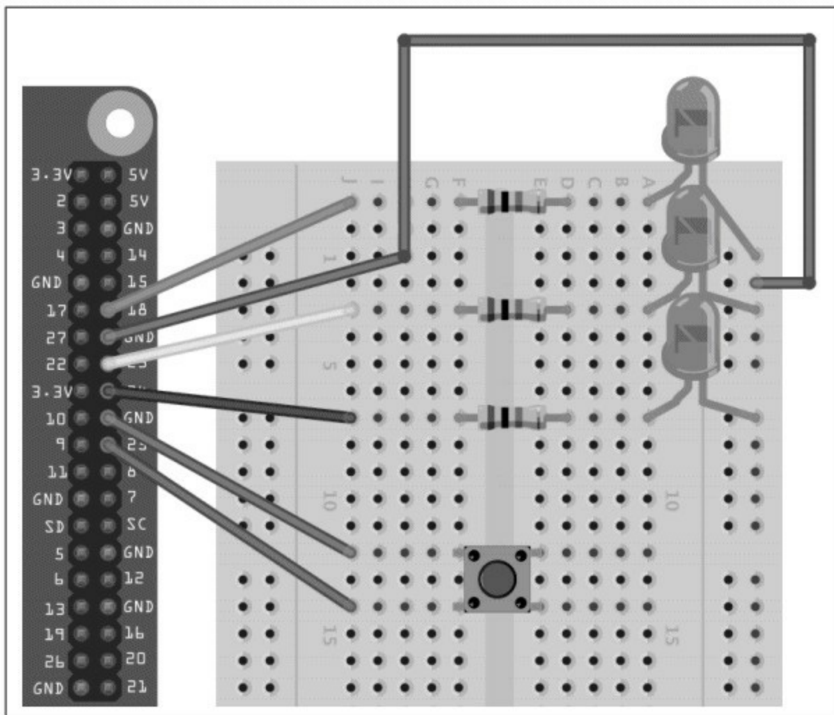
图15-1 利用网页控制GPIO输出时所用的面包板布局
