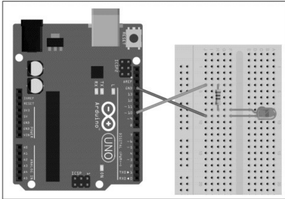
图16-5 Arduino和LED布线图
