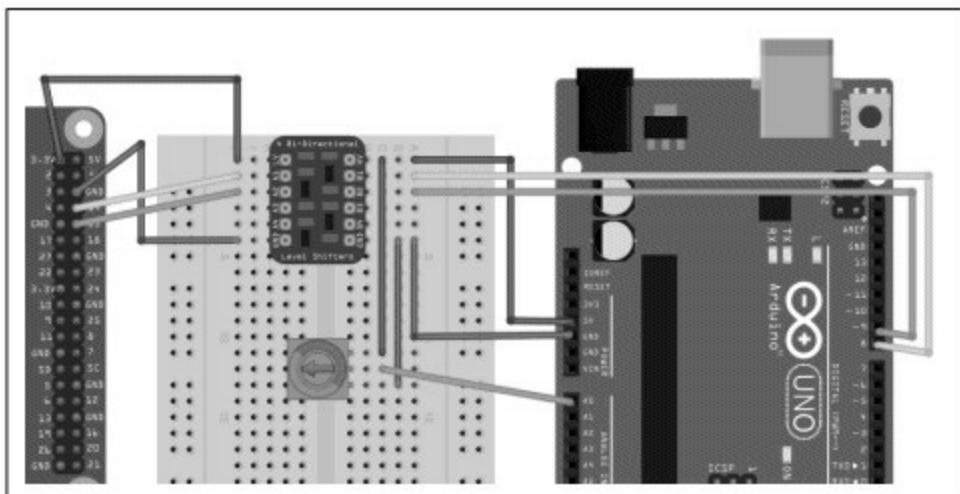
图16-14 Arduino串行通信布线图
