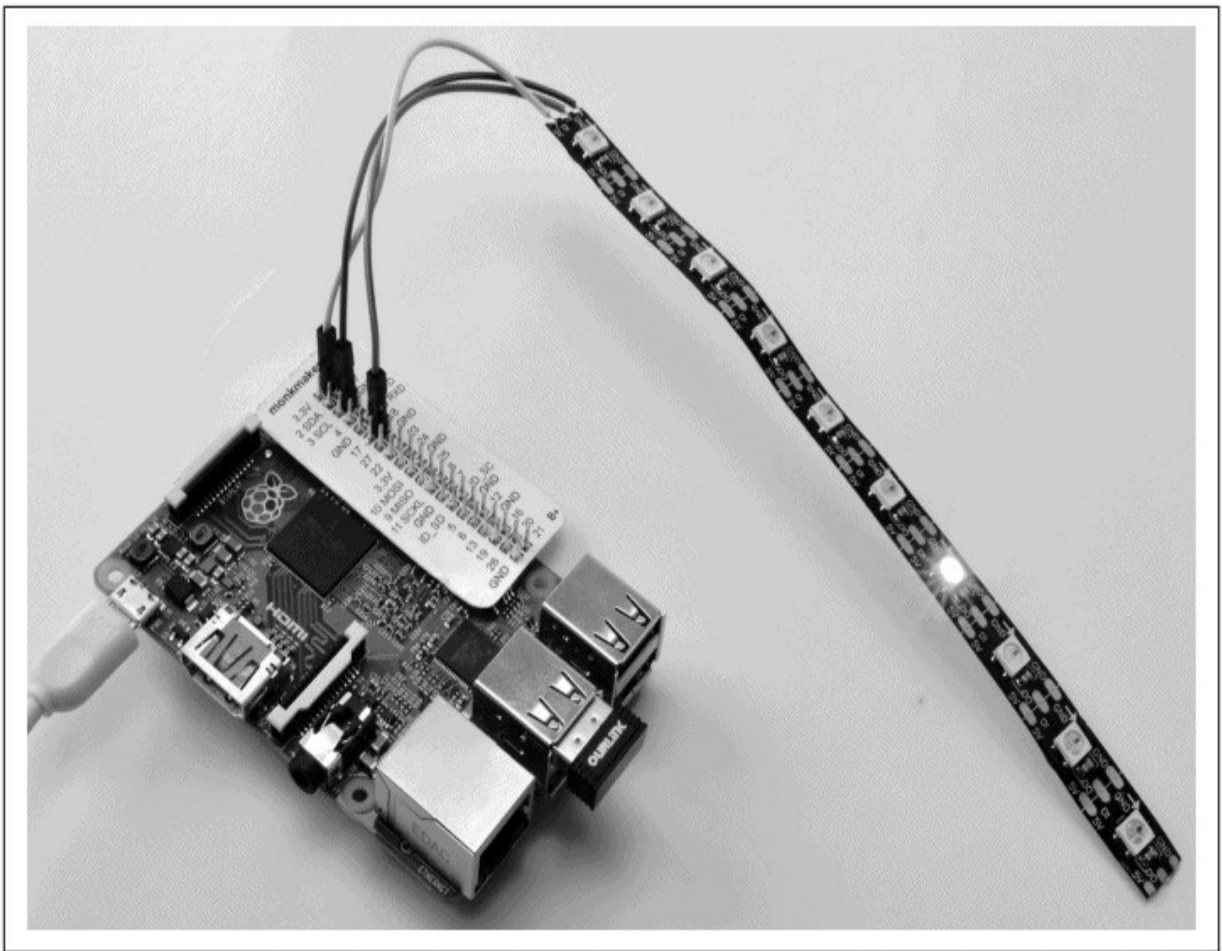
图14-8 具有10个LED的灯条
