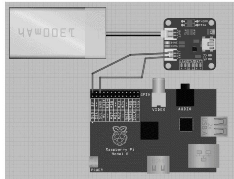
图9-18 利用3.7V锂电池为树莓派供电
