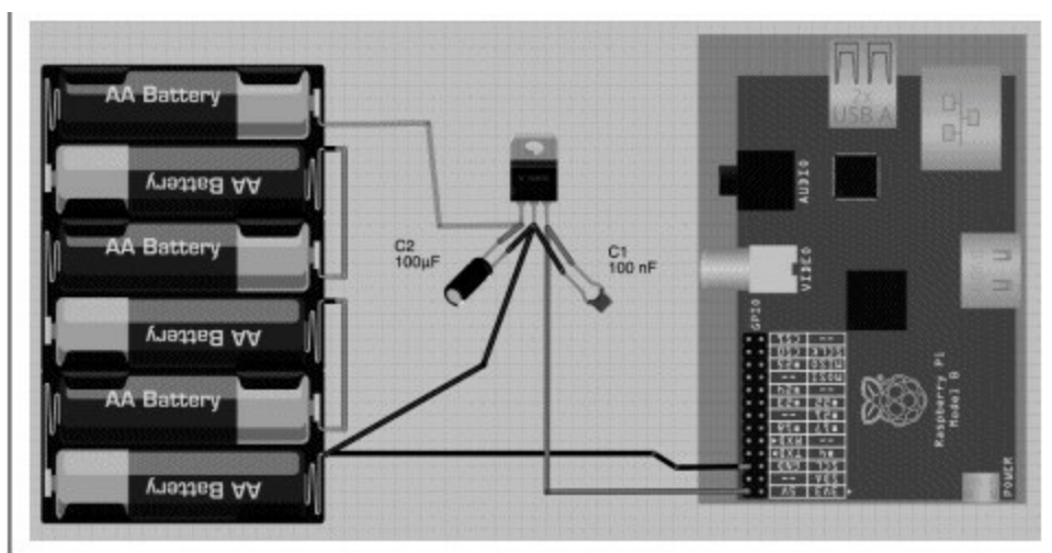
图9-16 利用AA电池为树莓派供电
