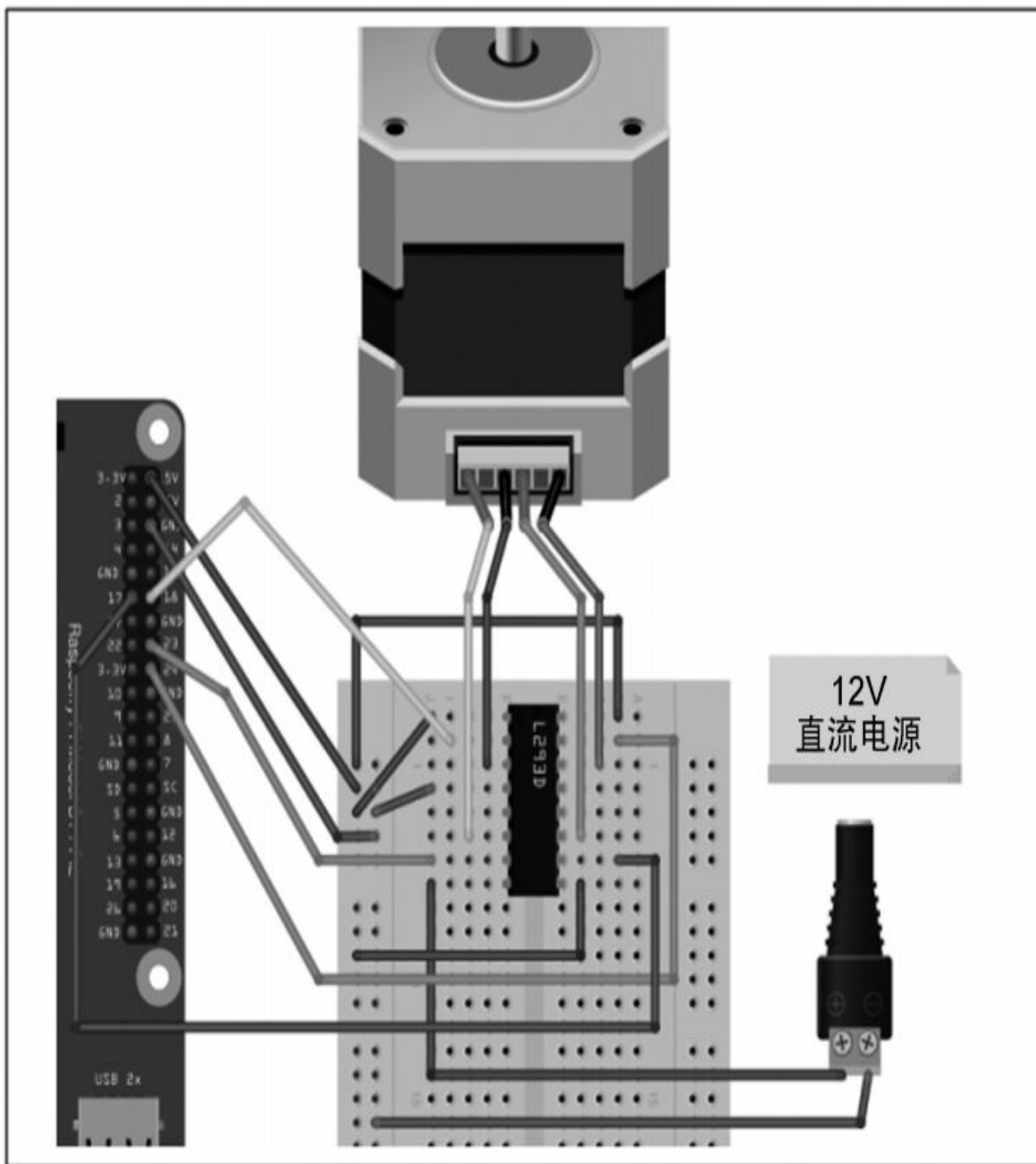
图11-14 使用L293D控制双极步进电机
