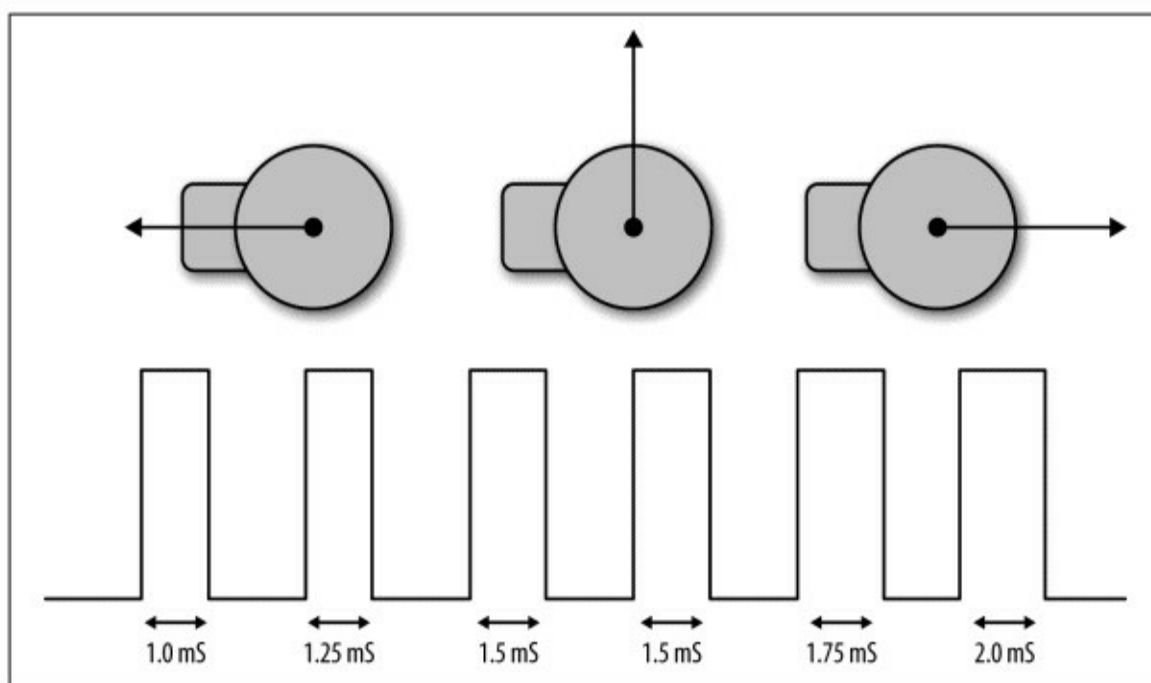
图11-4 伺服电机
