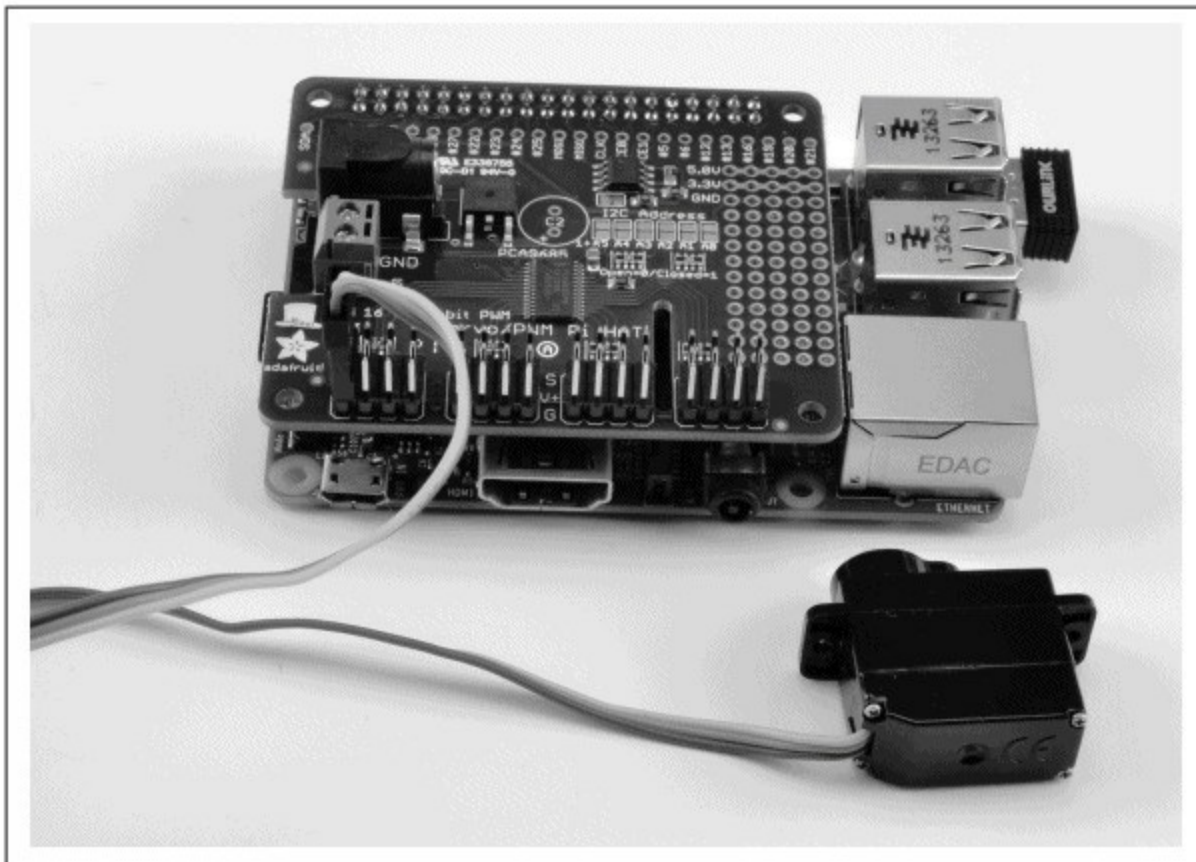
图11-5 Adafruit的伺服电机HAT
