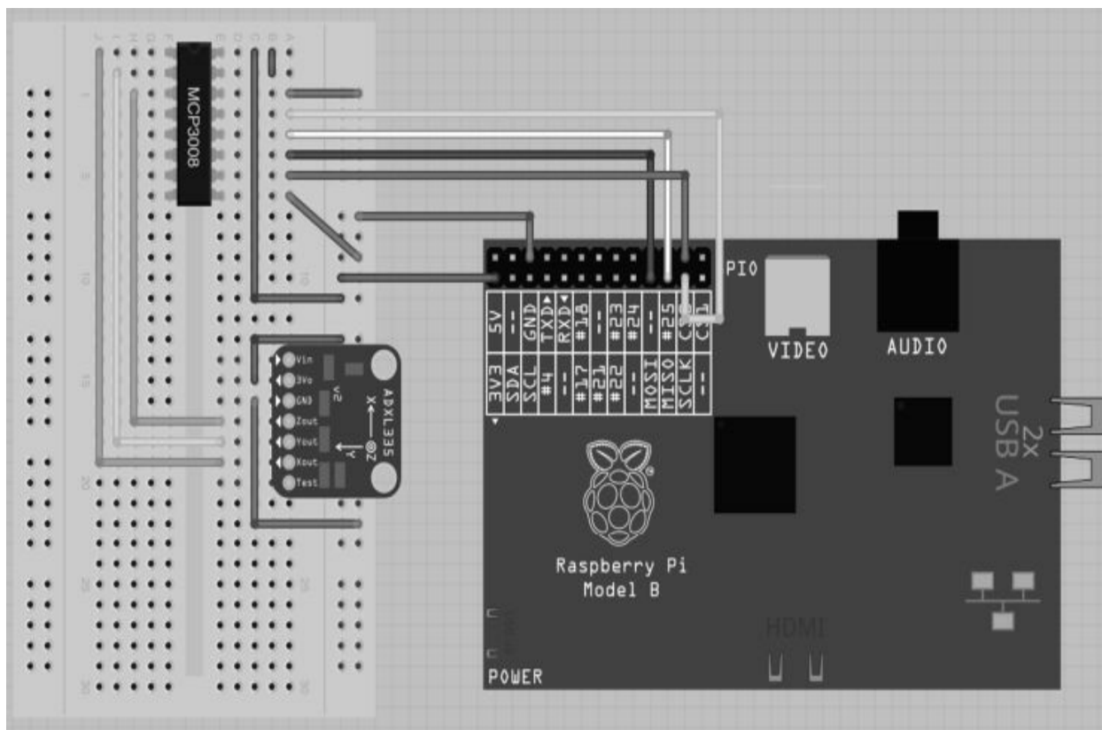
图13-18 使用三轴加速度计
