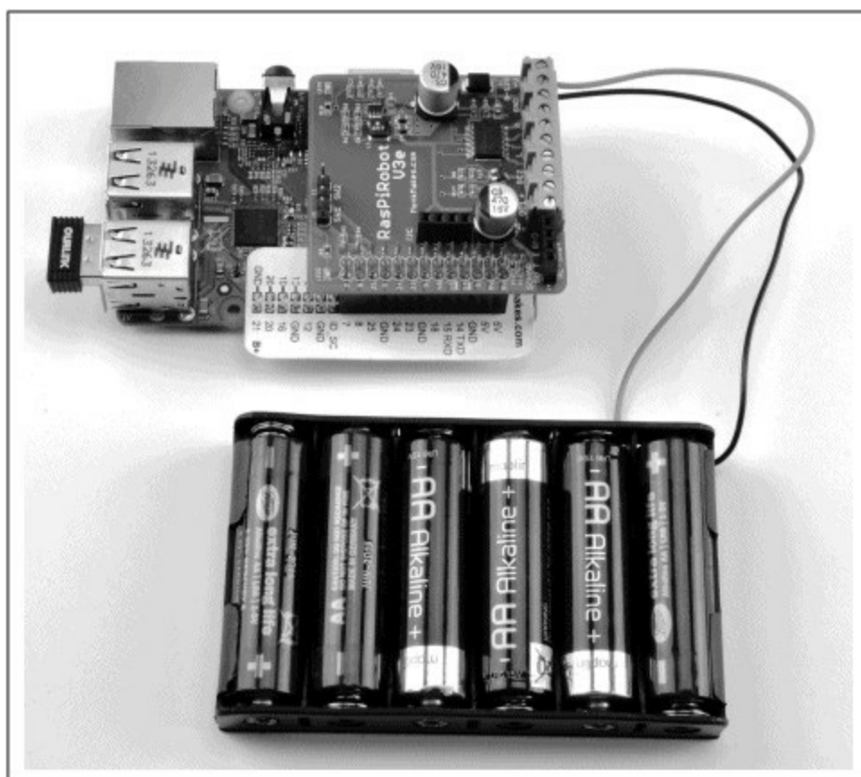
图9-17 利用RasPiRobot Board V3为树莓派供电
