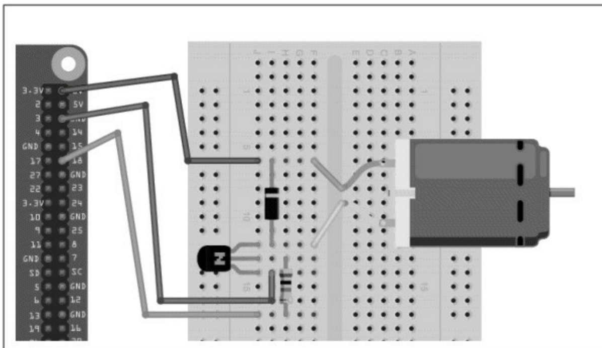
图11-7 控制低功率电机
