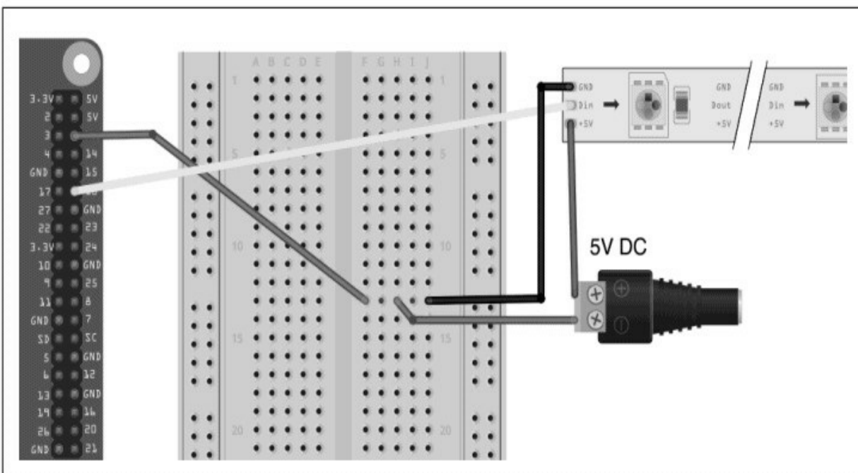
图14-10 利用外部电源为LED灯条供电
