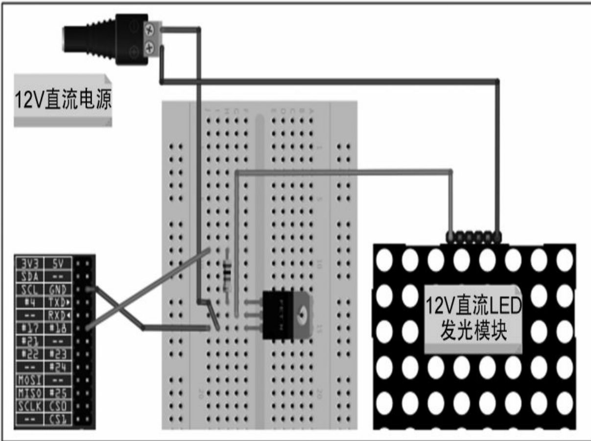
图10-4 利用MOSFET控制大电流
