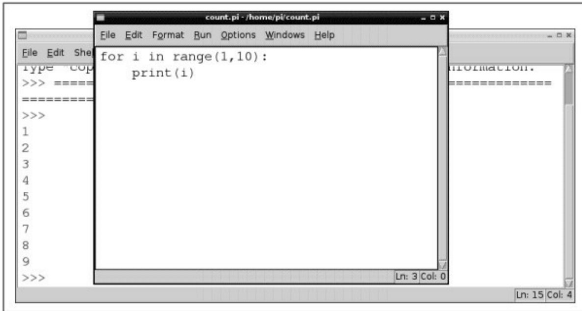
图5-3 IDLE编辑器
