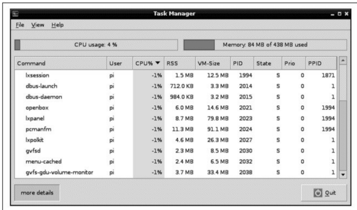
图3-8 任务管理器
