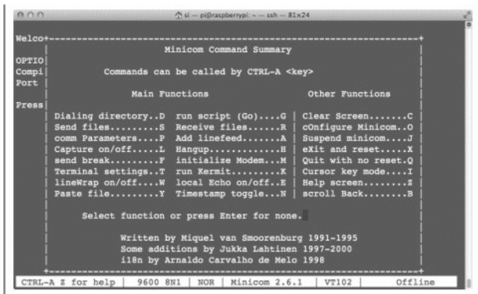
图9-8 Minicom命令
