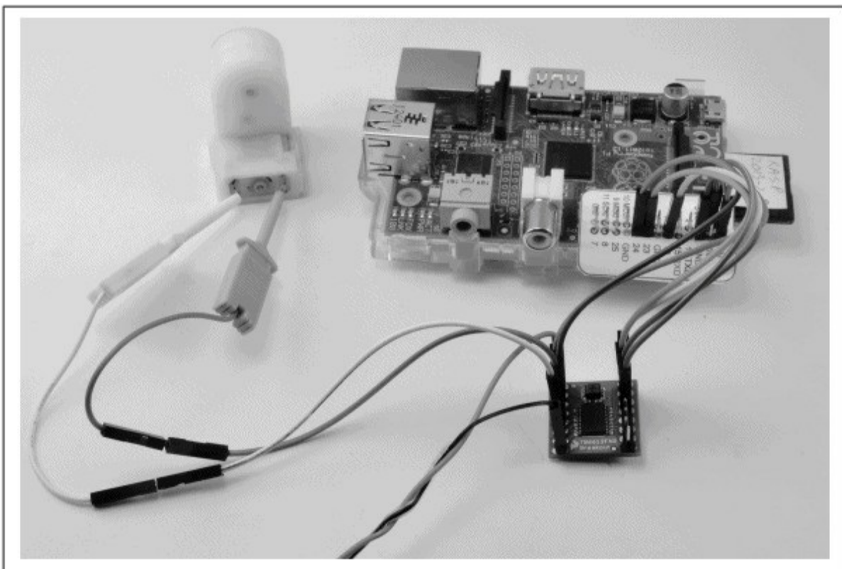
图11-10 使用SparkFun电动机控制器和齿轮减速电机
