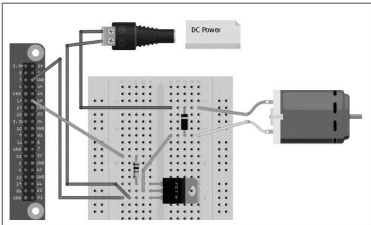
图11-6 控制高功率电机
