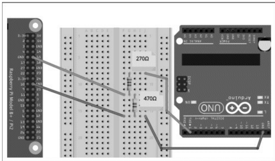
图9-14 利用电阻将5V信号转换为3.3V
