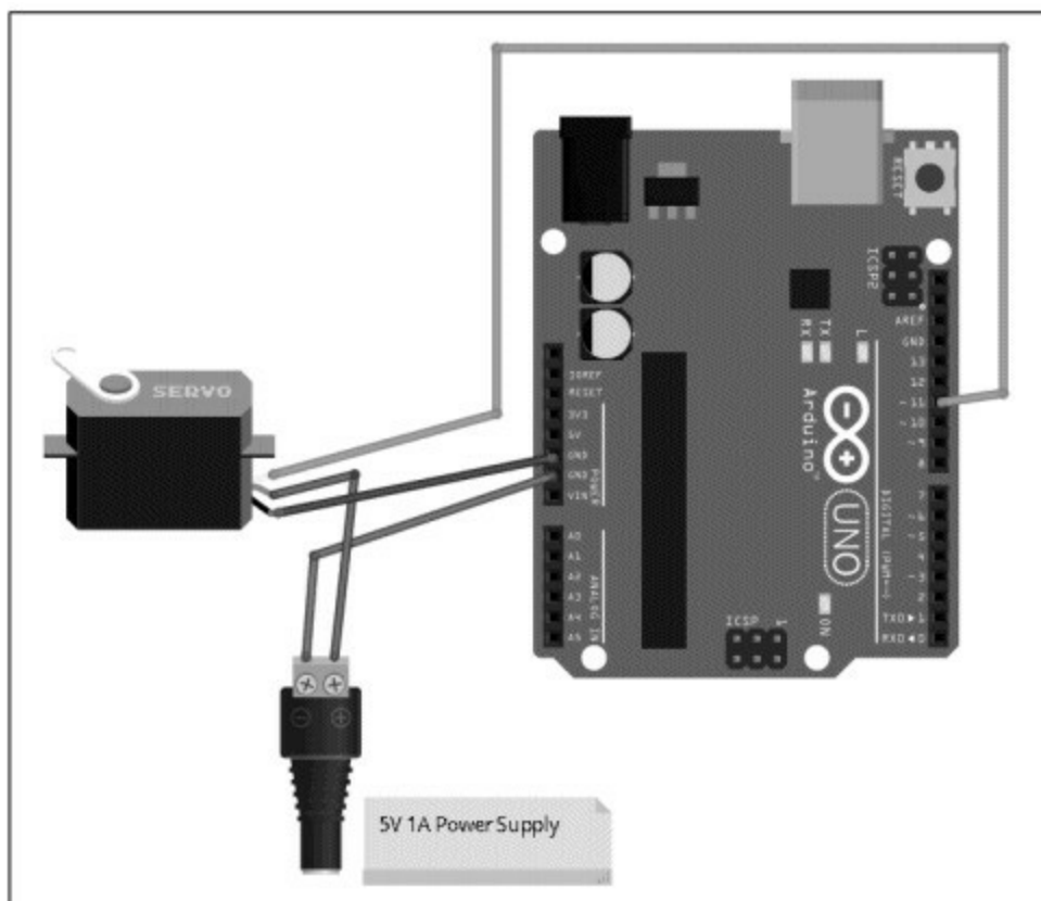
图16-13 Arduino控制伺服电机所需布线图
