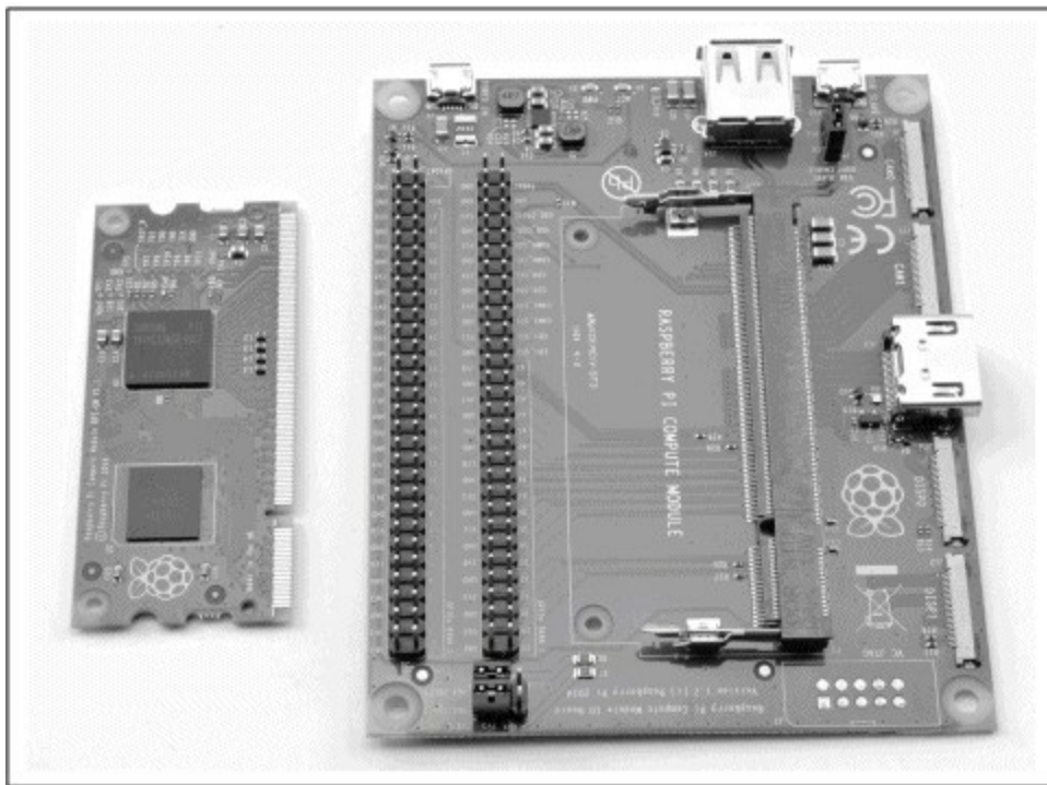
图9-29 树莓派的计算模块及其IO板
