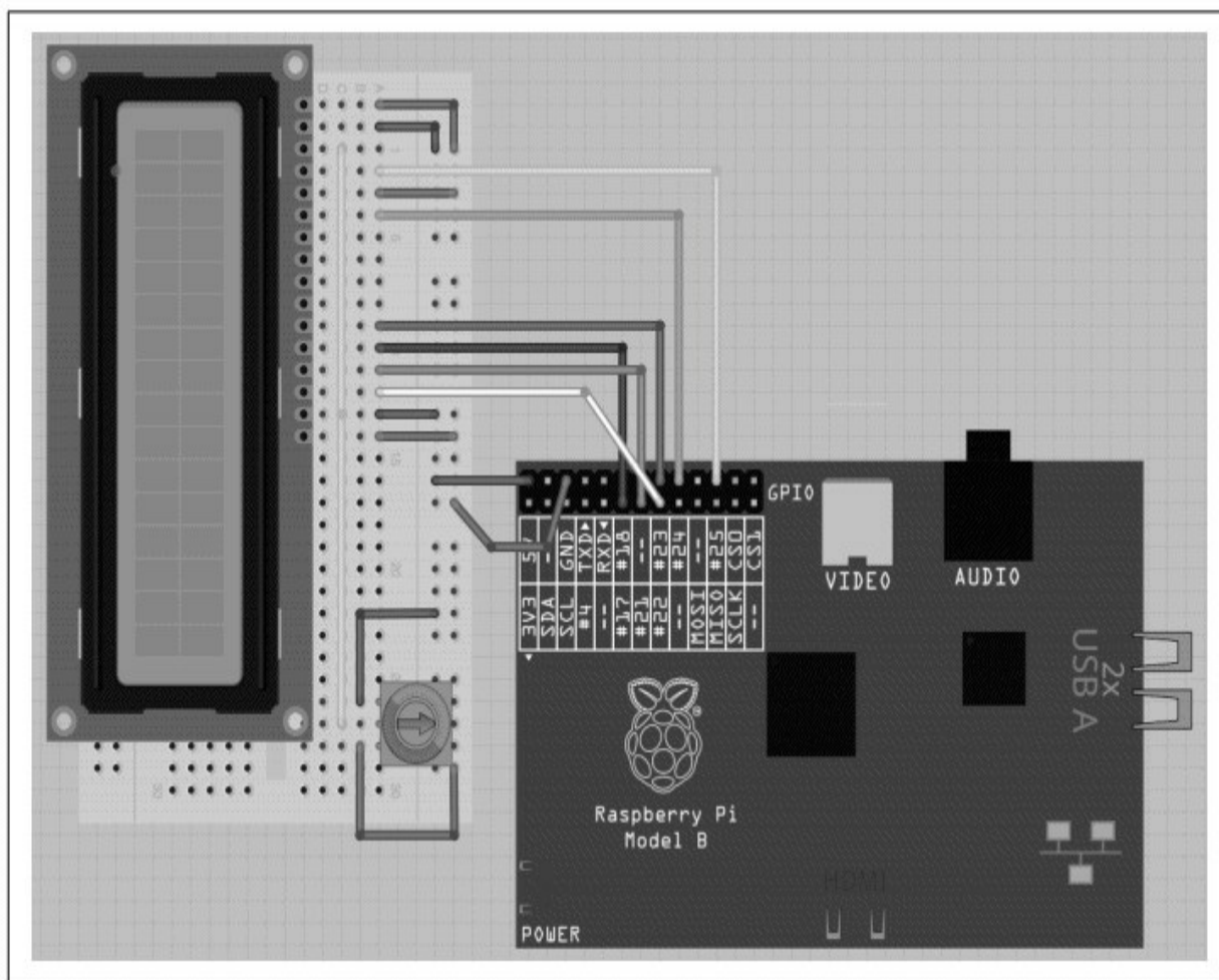
图14-6 将LCD显示设备连接至树莓派
