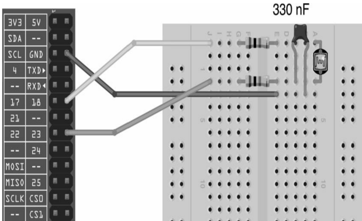
图13-4 利用树莓派测量光强
