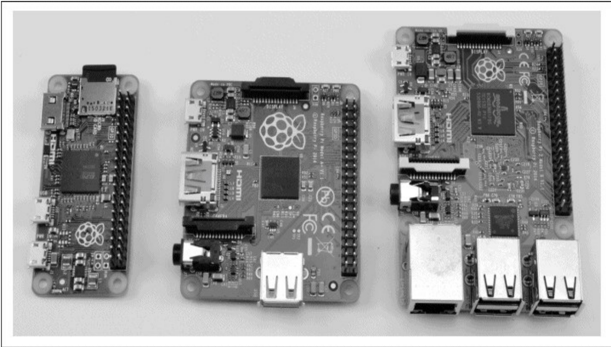
图1-1 Pi Zero（左）、A+型（中）和B型（右）树莓派2
