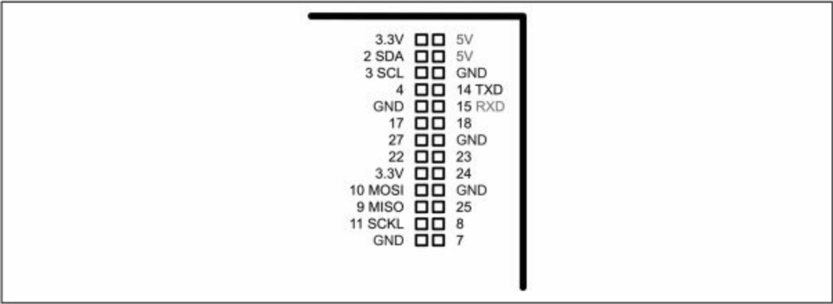
图B-2 B型树莓派第二版与A型树莓派的GPIO引脚
