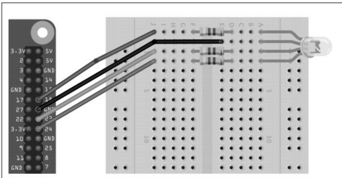
图10-10 在树莓派上使用RGB LED
