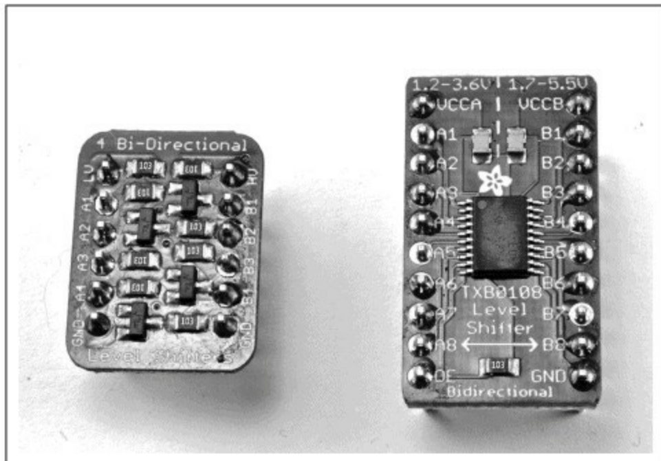
图9-15 电平转换模块进一步探讨
