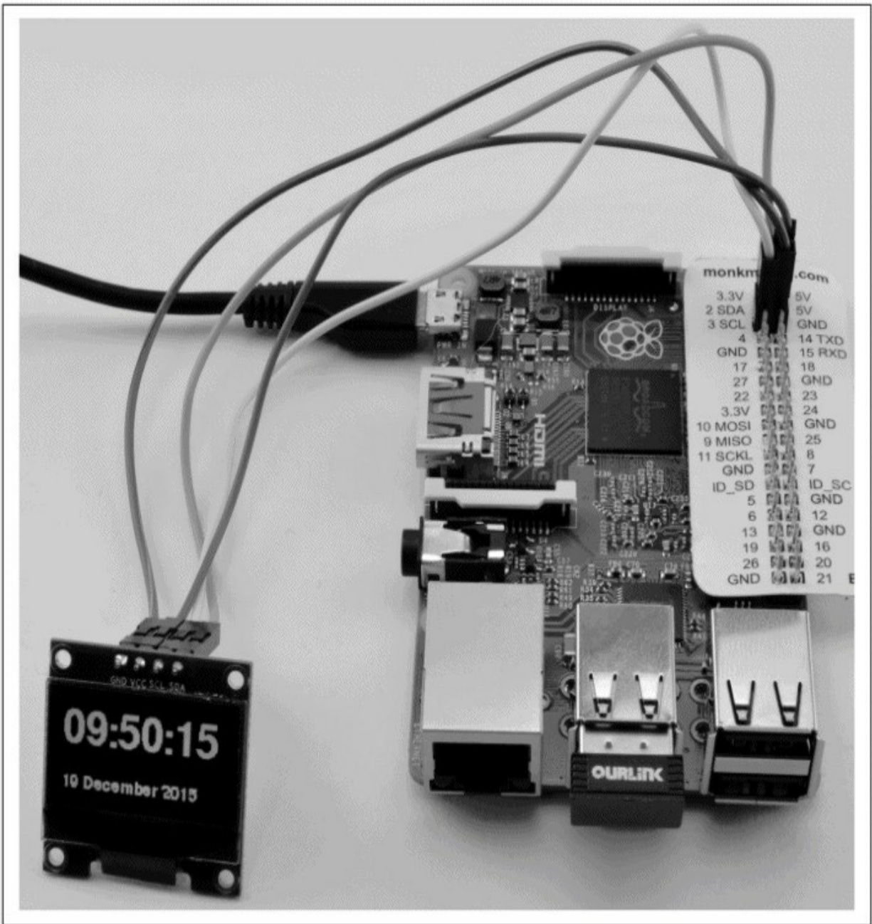
图14-7 I2C OLED显示器
