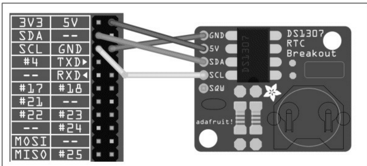
图12-18 连接RTC模块
