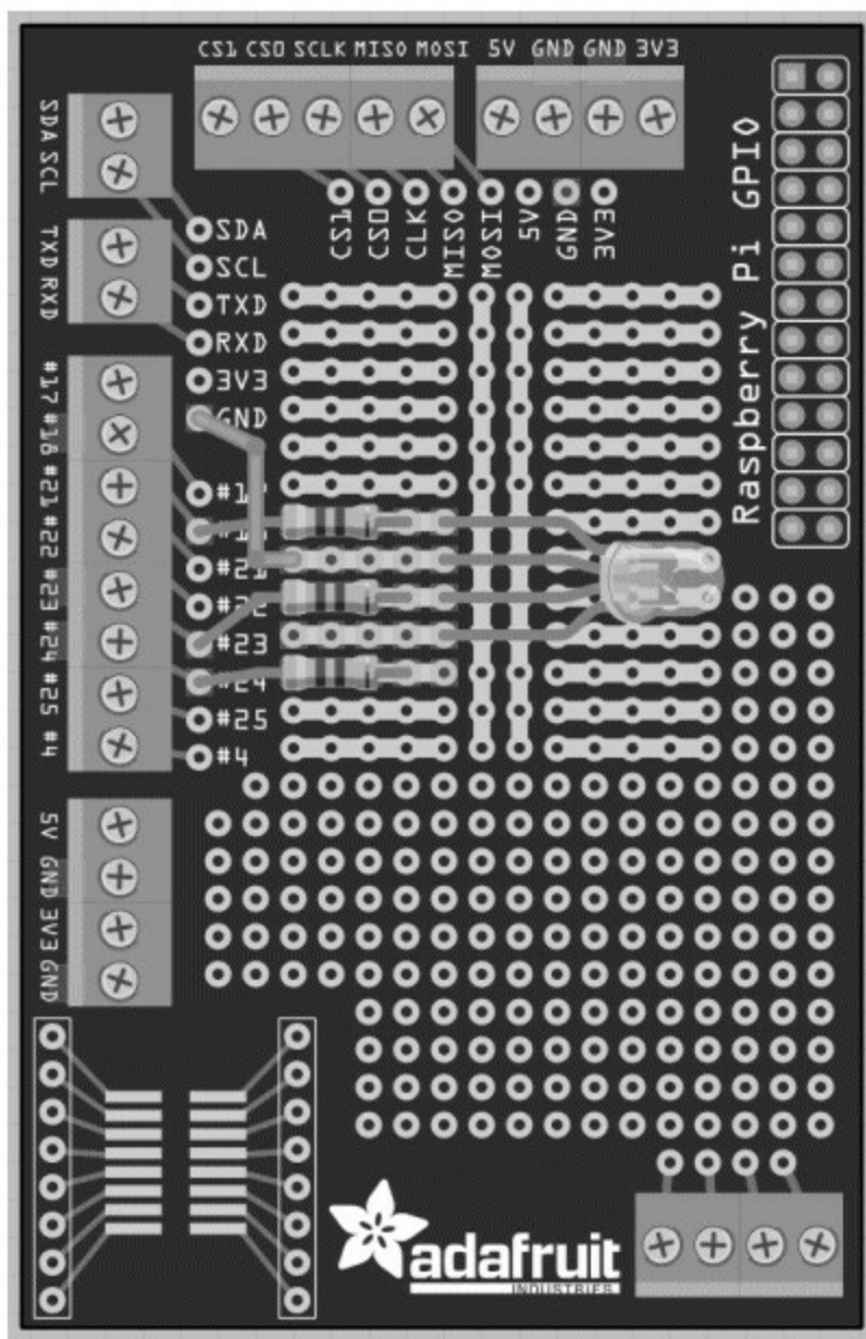
图9-23 Pi Plate上面的RGB LED的版面布局
