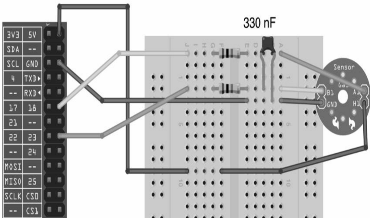
图13-9 将气体传感器连接至树莓派（直接连接）
