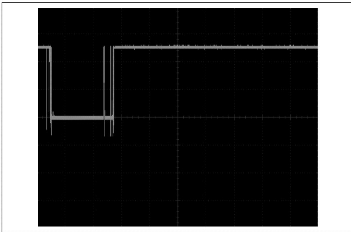
图12-8 廉价开关的触点抖动
