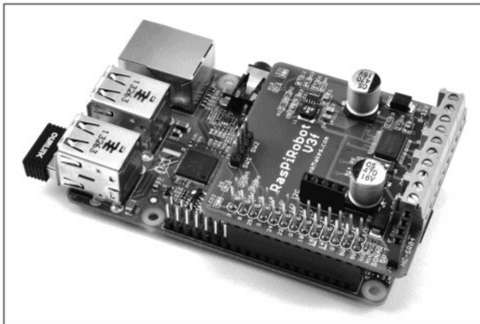
图9-21 RaspiRobot板 V3
