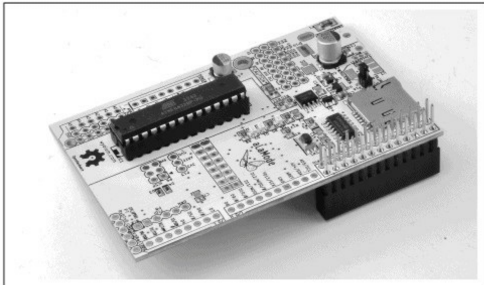
图16-18 aLaMode接口板
