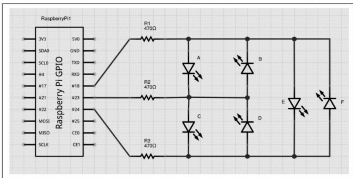
图10-12 Charlieplexing技术
