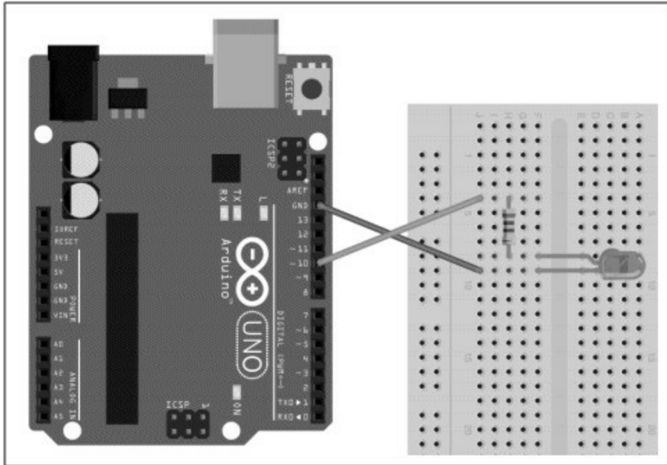
图16-11 利用Arduino的PWM控制LED的布线图
