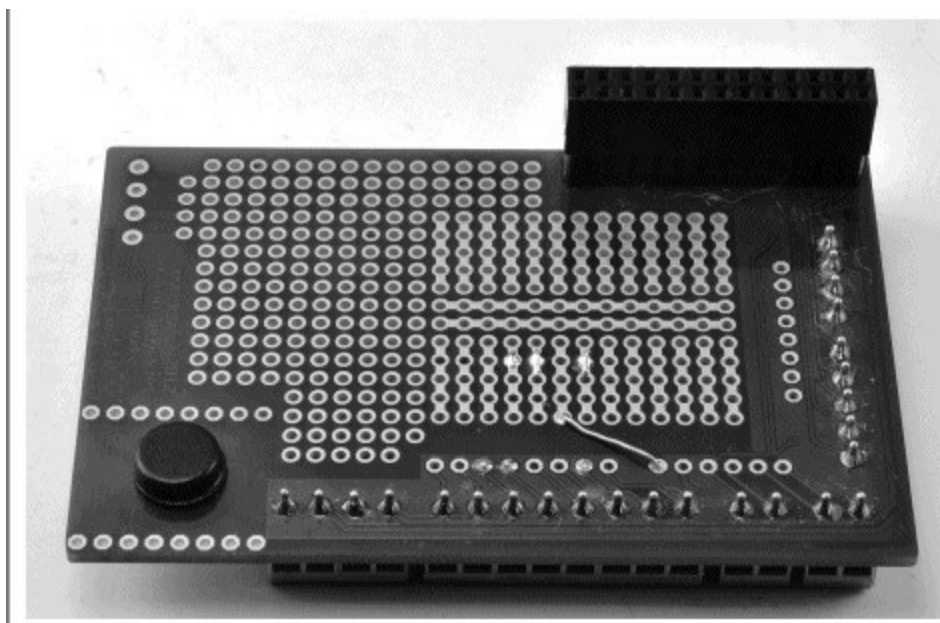
图9-26 焊接连接Pi Plate的导线
