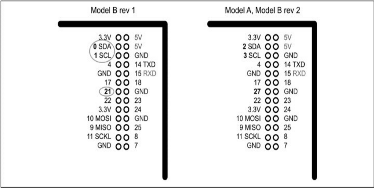
图9-1 GPIO引脚（26针）
