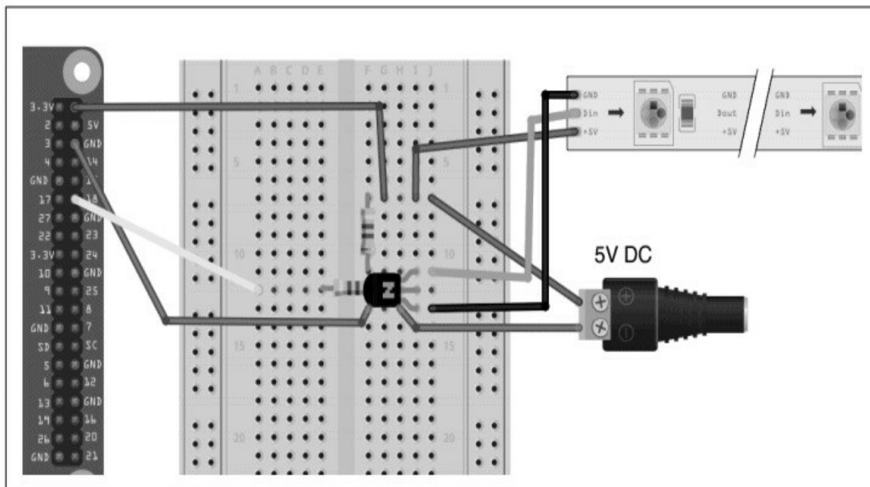
图14-11 使用逻辑电平变换器
