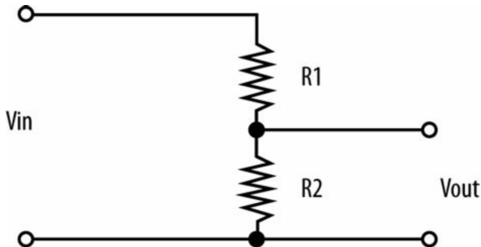
图13-13 分压器
