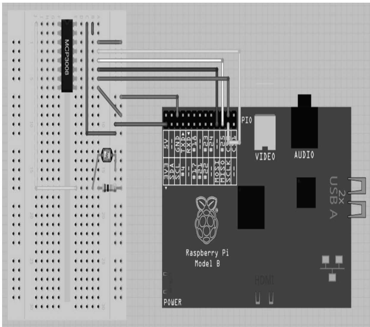
图13-14 使用光敏电阻器和ADC
