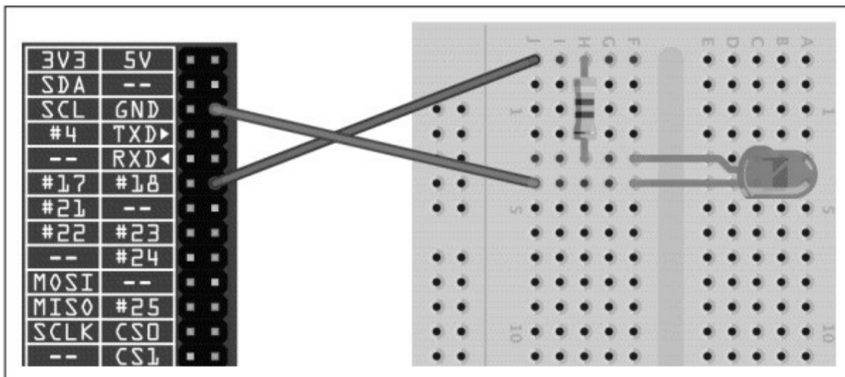
图10-1 将LED连接到树莓派上面
