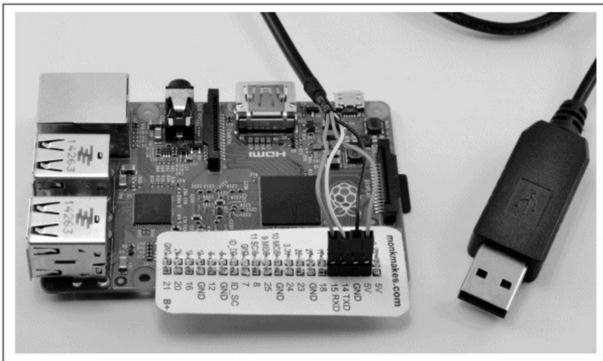
图2-5 控制台线
