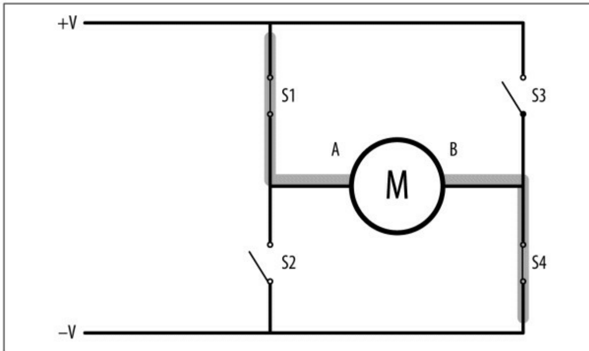
图11-11 H-Bridge
