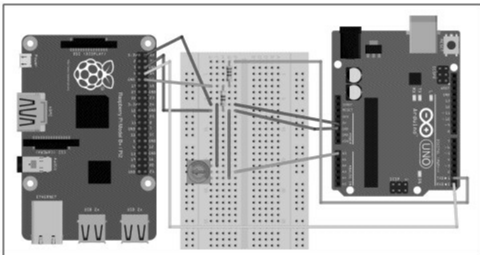
图16-15 Arduino（使用电阻）串行通信布线图
