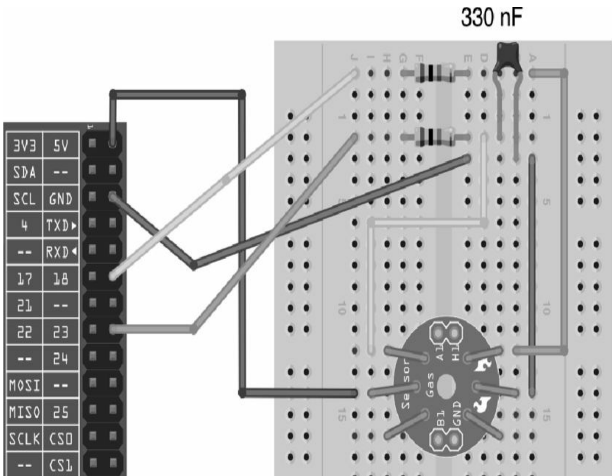
图13-8 将气体传感器连接到树莓派（分线板）
