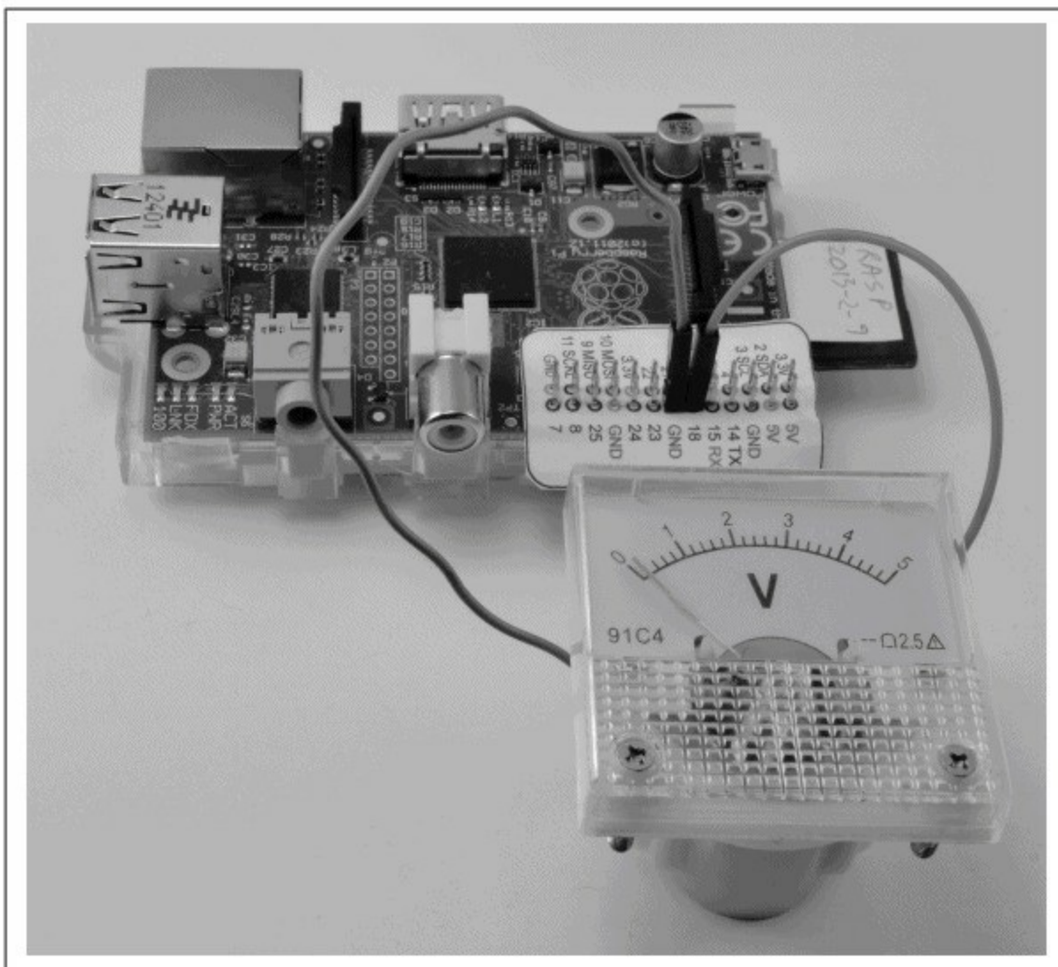
图10-14 直接将电压表连接至GPIO引脚
