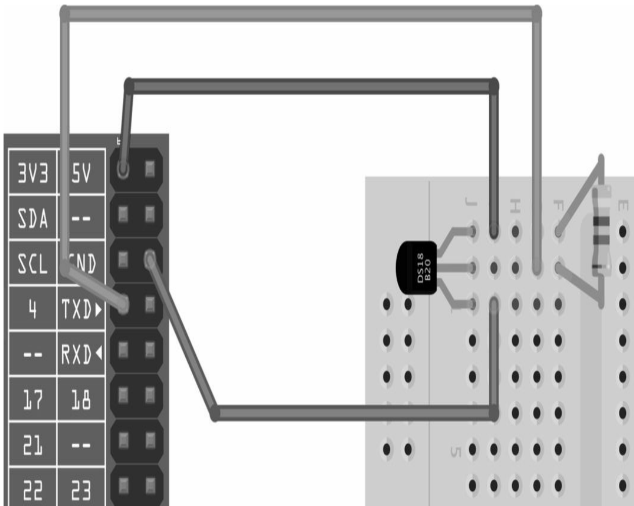
图13-17 将一个DS18B20连接到树莓派
