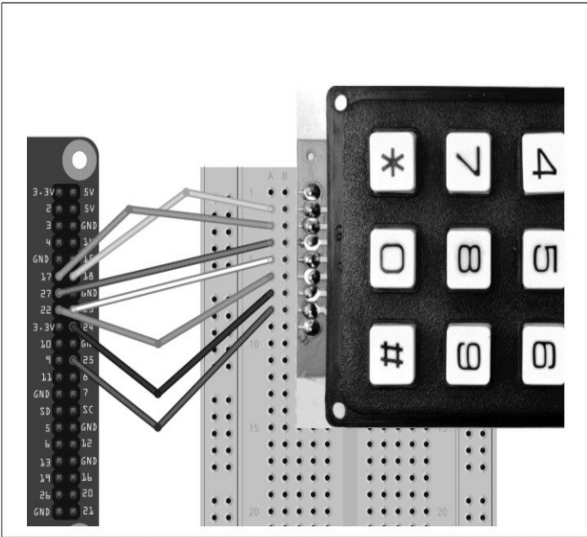
图12-12 数字键盘布线图
