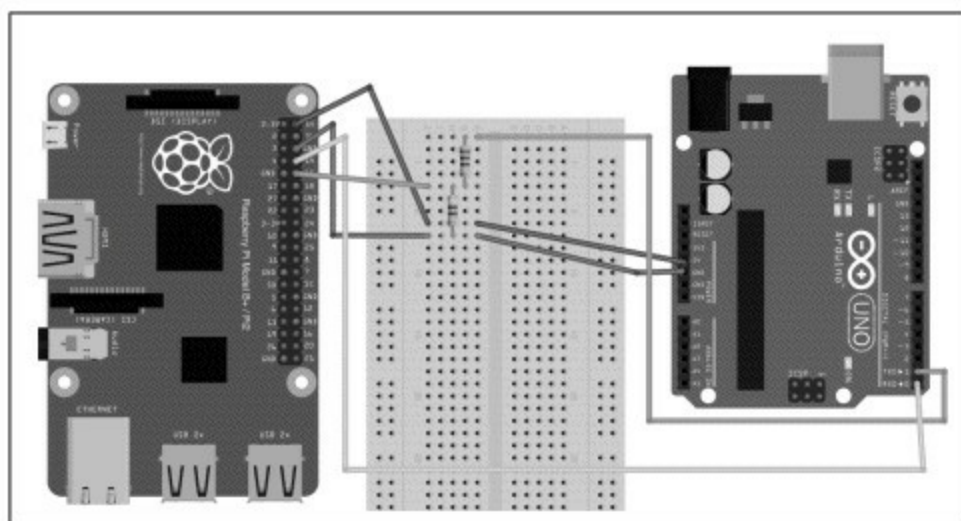
图16-8 将一对电阻器用于Arduino串行通信的布线图
