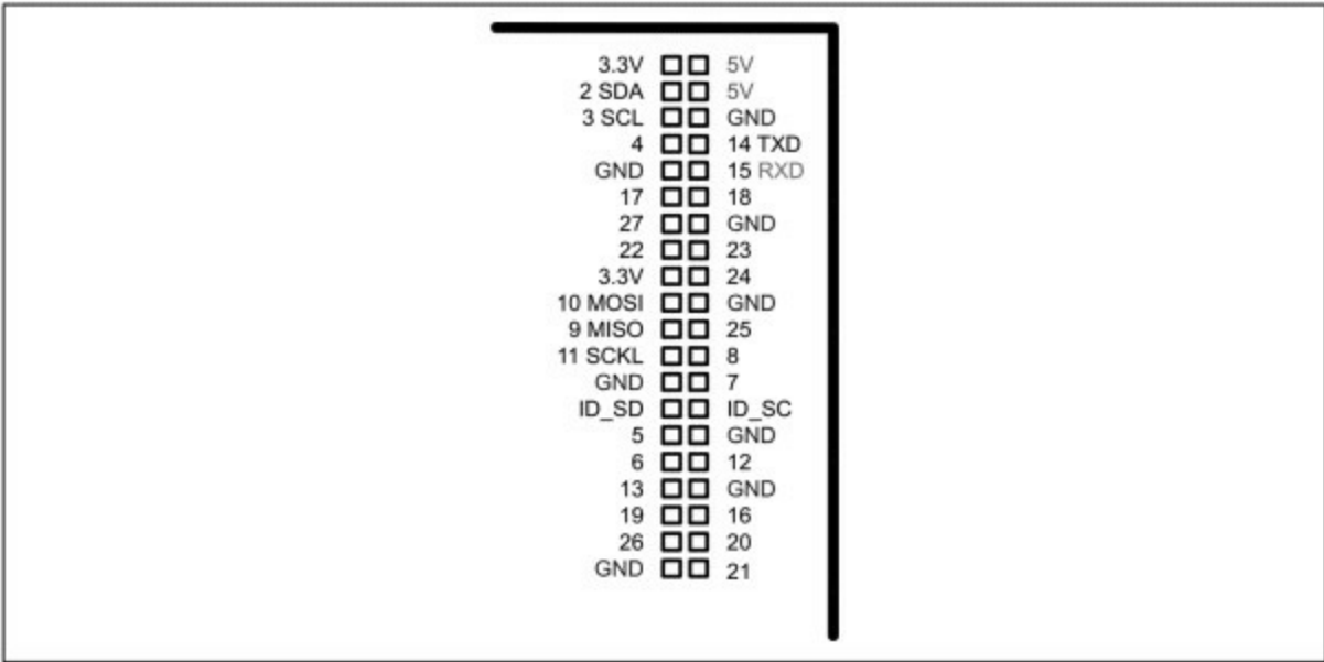
图B-1 40引脚树莓派的引脚
