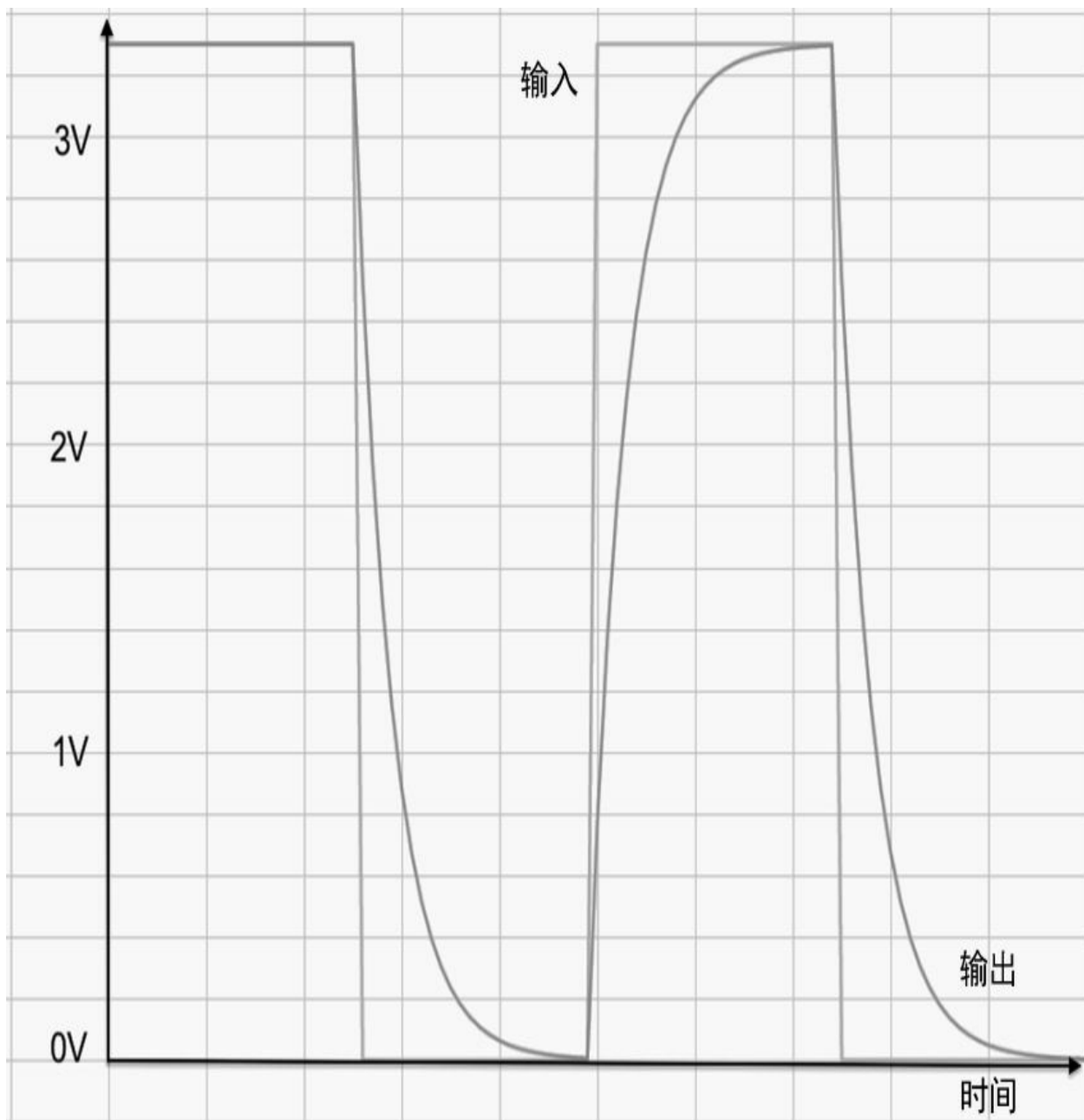
图13-3 电容器的充电和放电参考资料
