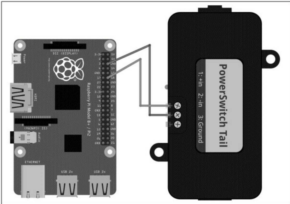
图10-7 在树莓派上使用PowerSwitch Tail
