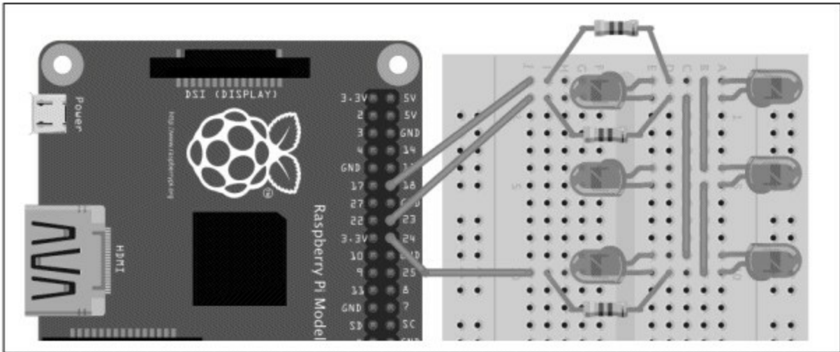
图10-13 Charlieplexing技术所用面包板的布局
