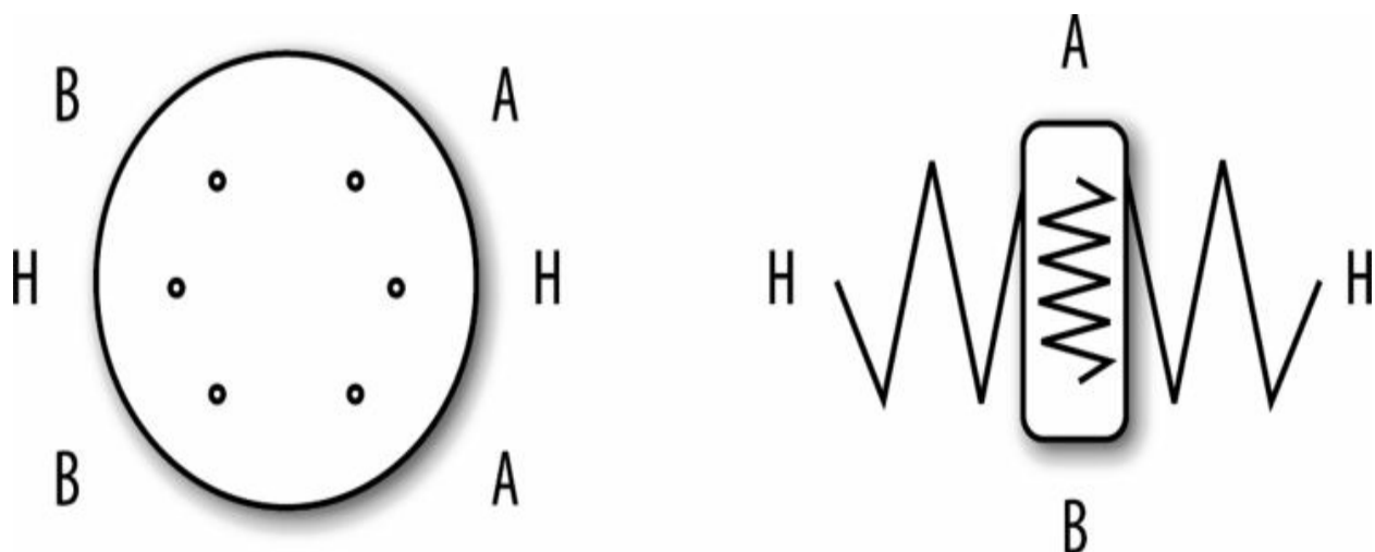
图13-10 甲烷气体传感器
