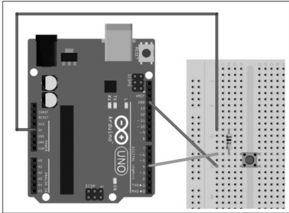
图16-9 Arduino与按钮开关的布线图
