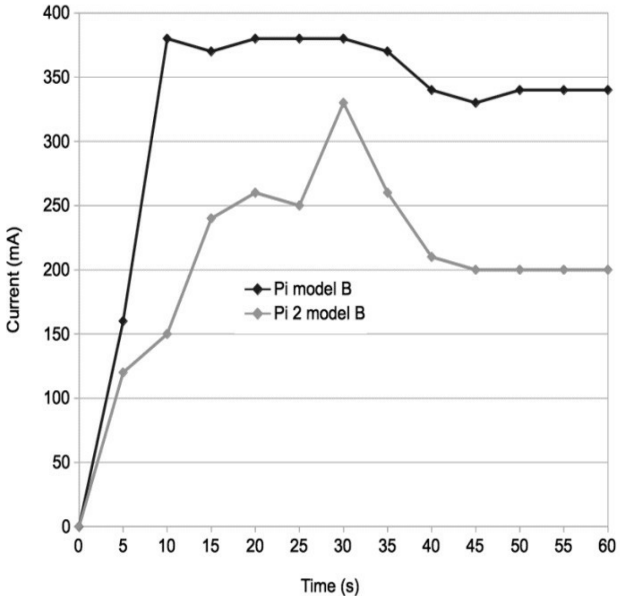
图1-3 树莓派在引导期间的电流消耗量
