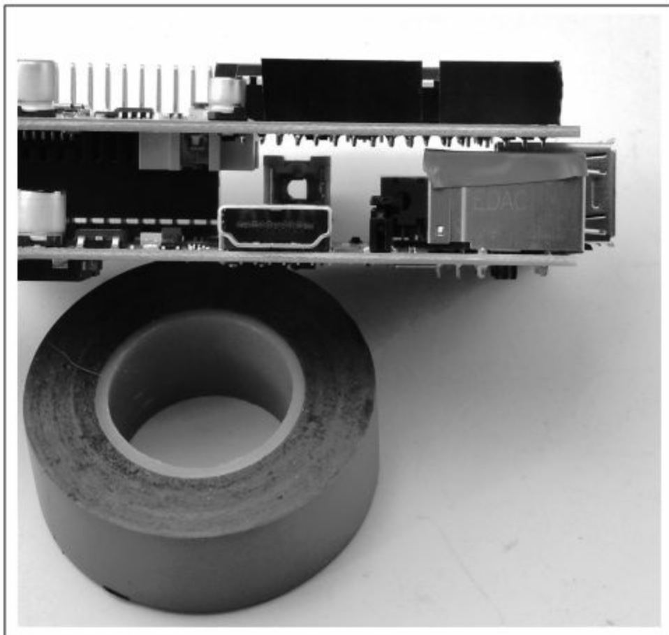
图16-20 为树莓派RJ45接口进行绝缘处理
