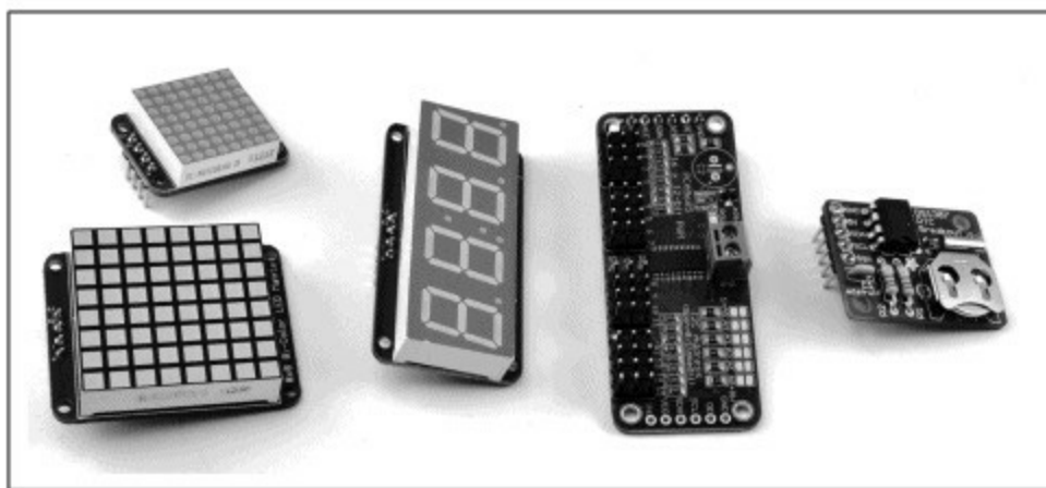
图9-6 I2C模块
