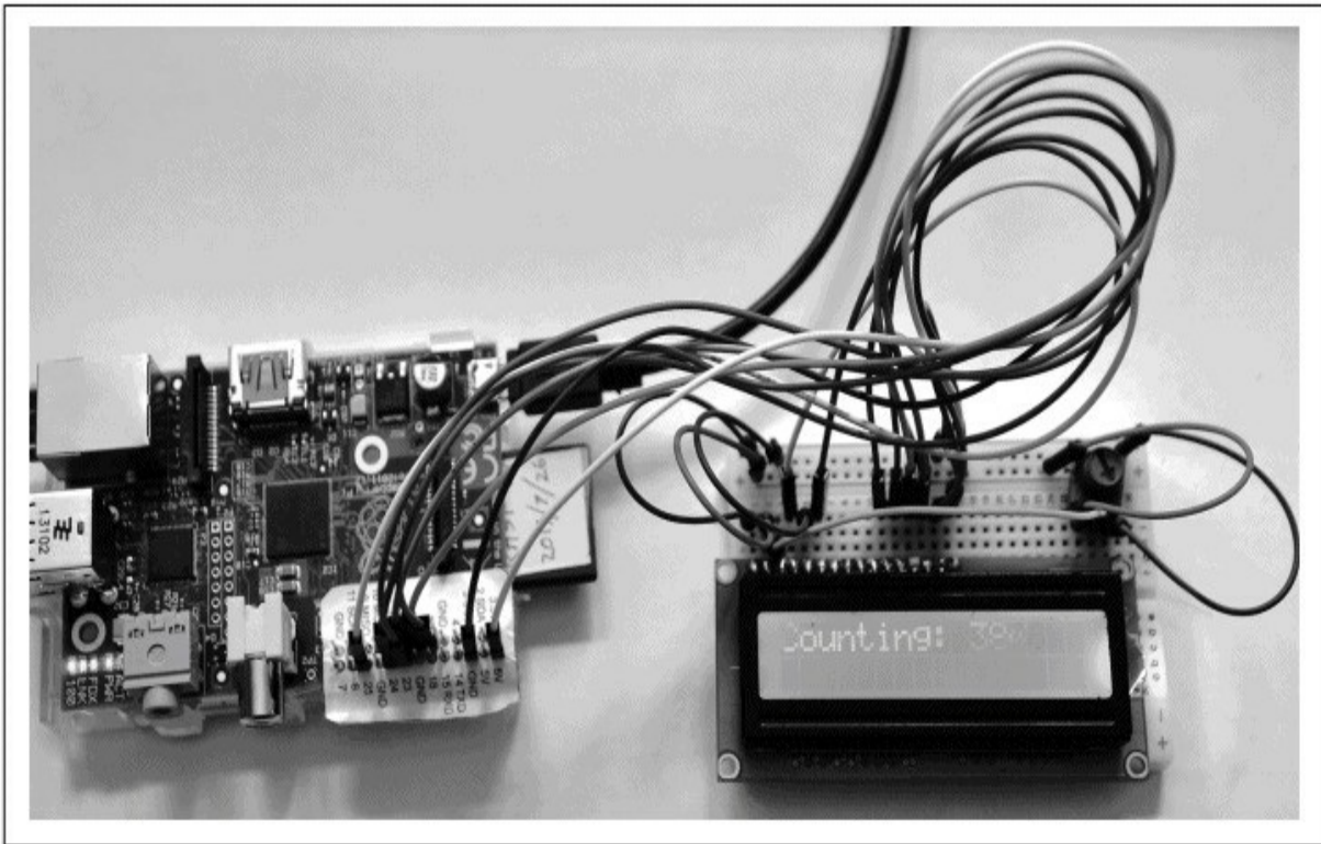
图14-5 连接到树莓派上面的一个16×2LCD显示设备
