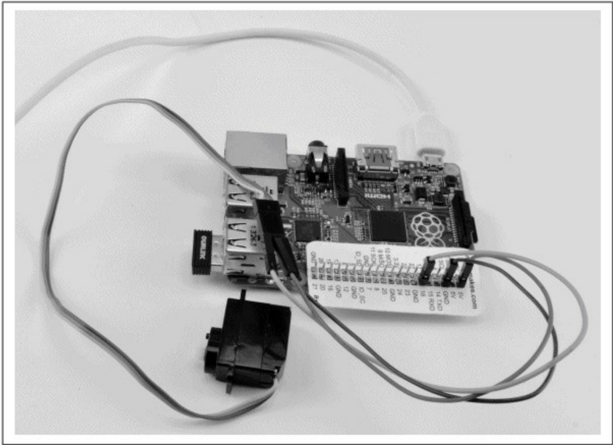
图11-1 将小型伺服电机直接连接到树莓派B+
