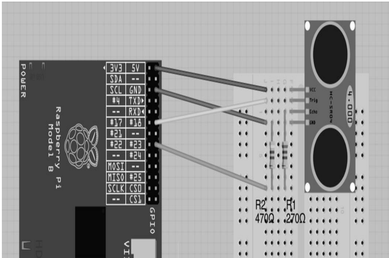
图13-23 将SR-04测距仪连接至树莓派
