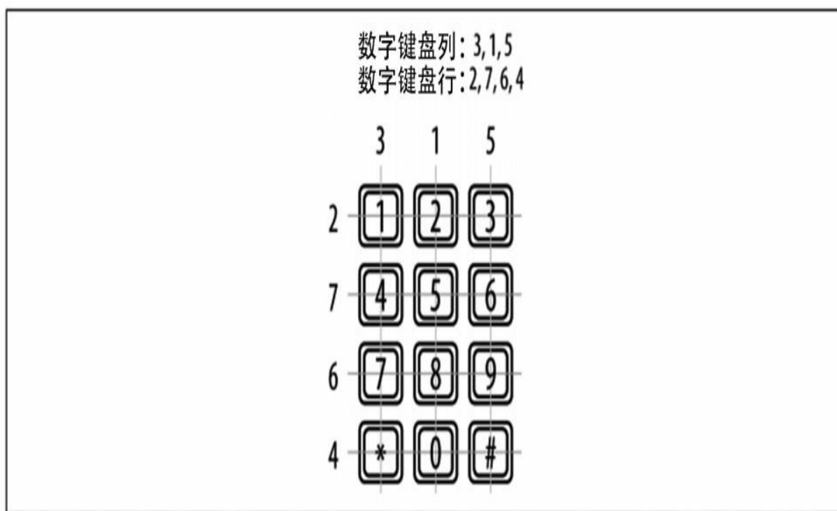
图12-13 数字键盘引脚的连接
