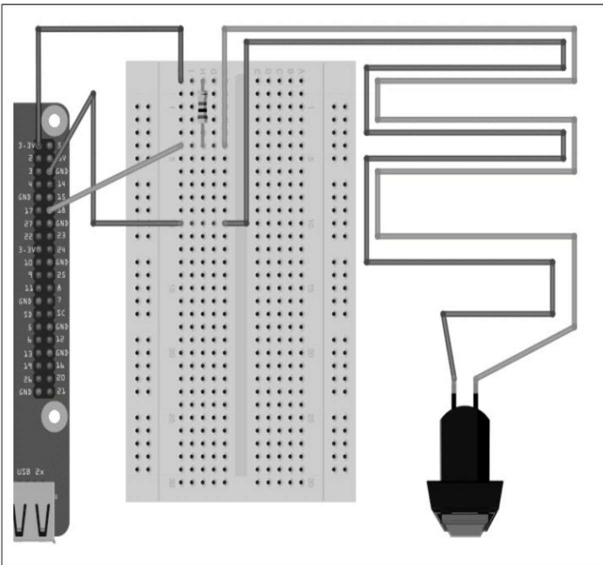
图12-9 使用外部上拉电阻
