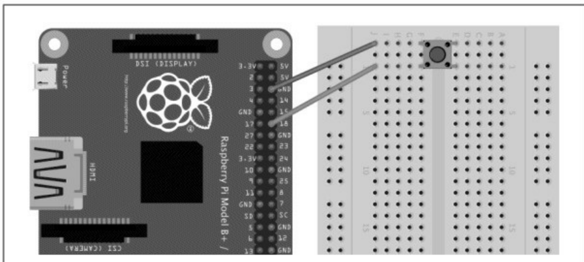
图10-16 将开关连接至GPIO输入来演示中断
