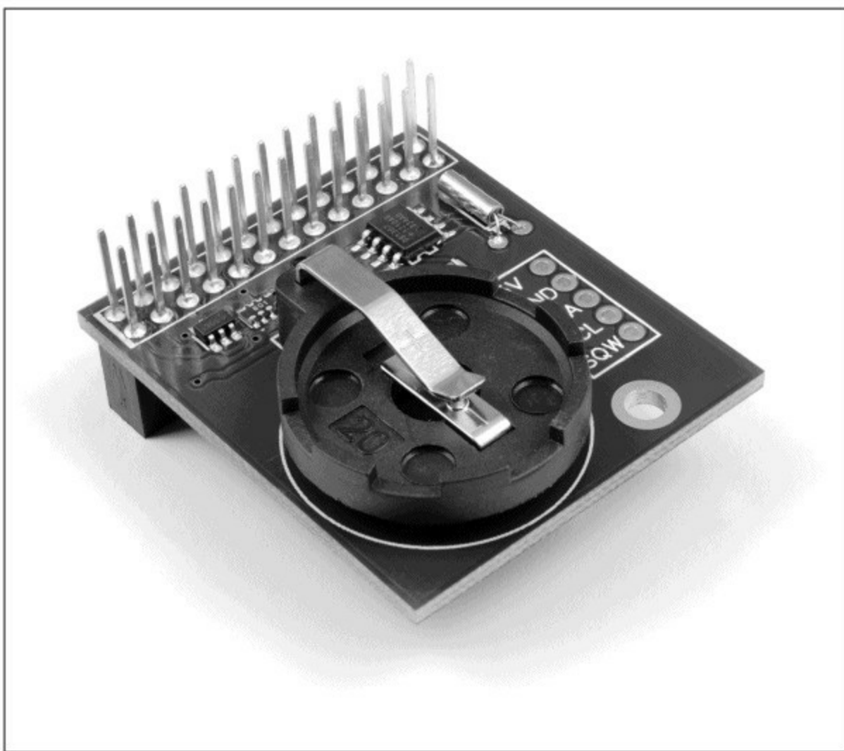
图12-19 AB Electronics的RTC模块
