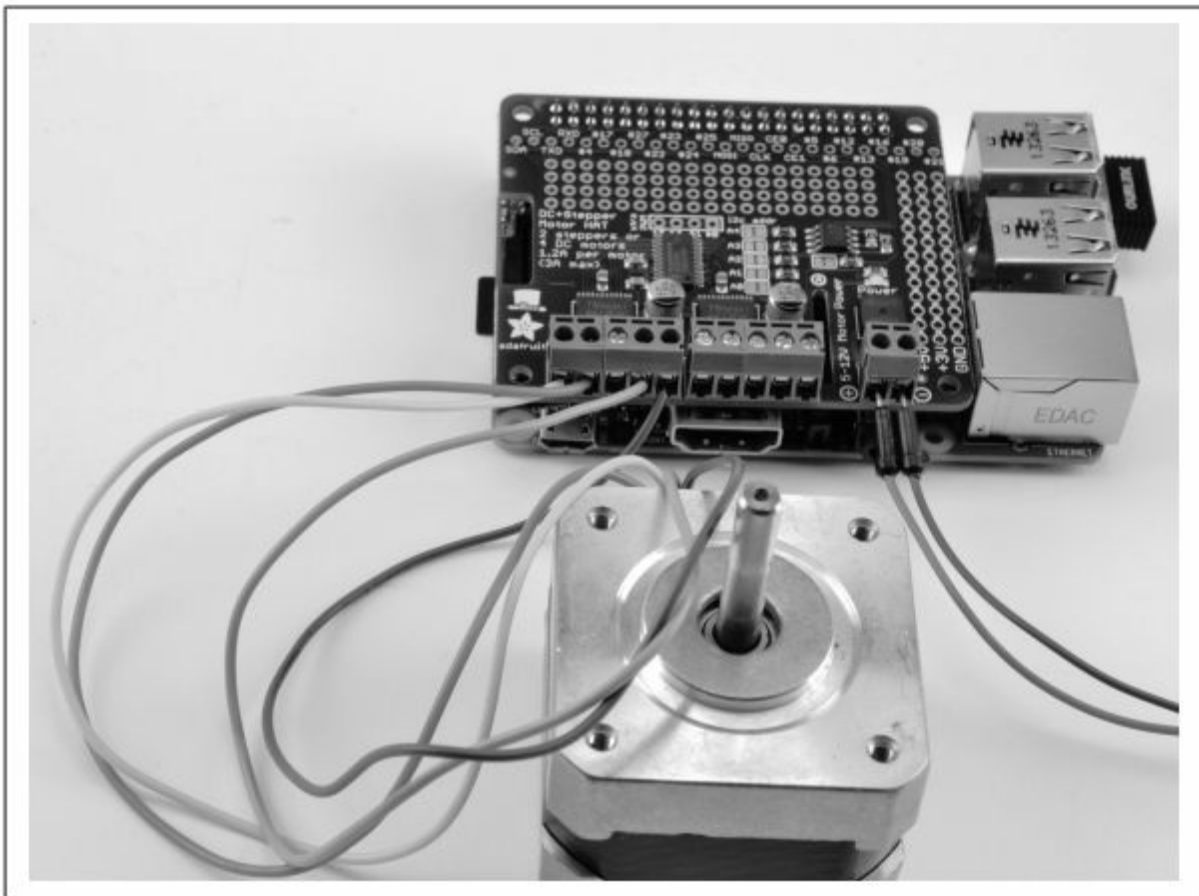
图11-15 使用Adafruit的步进电机HAT控制双极步进电机
