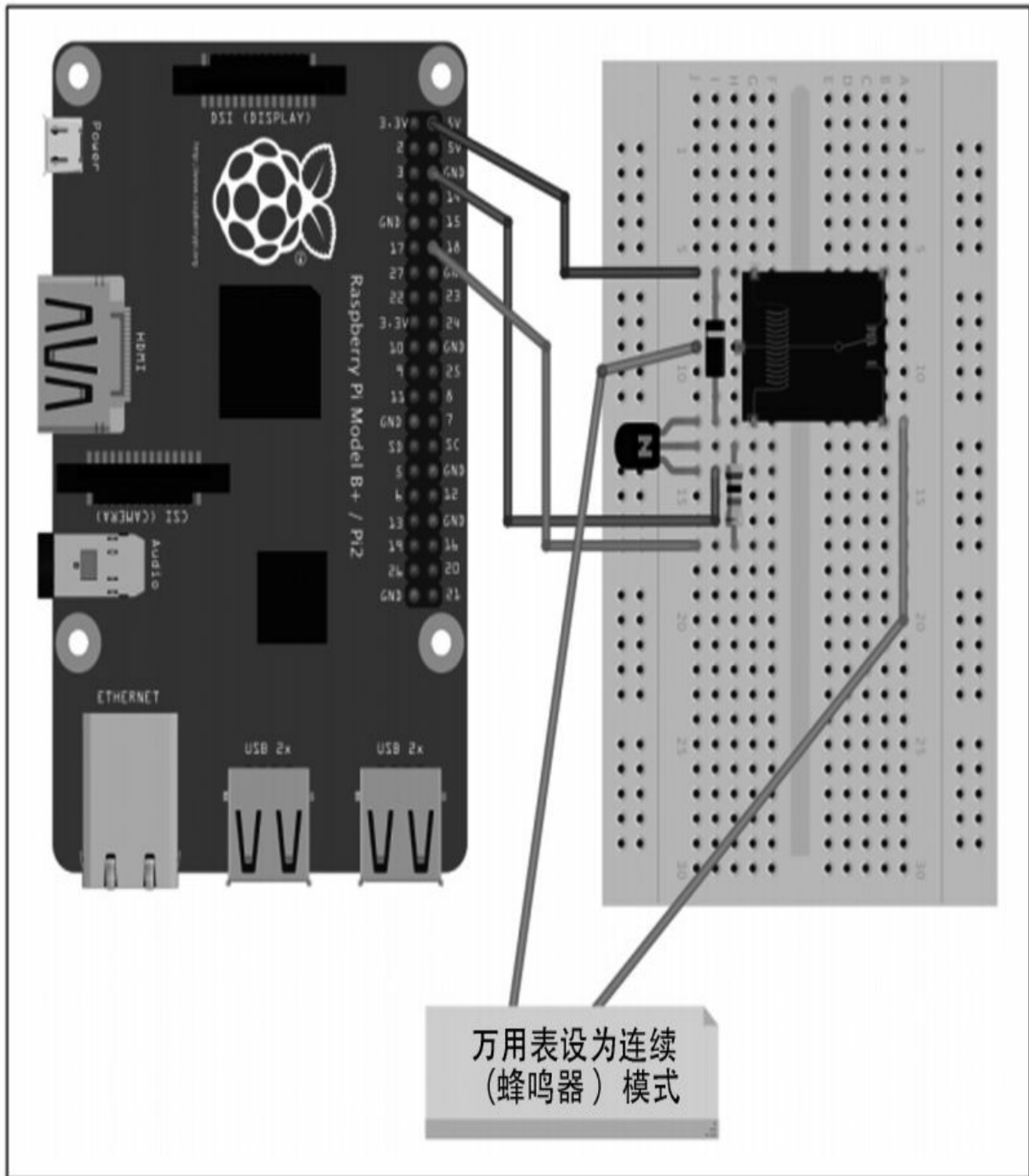
图10-5 使用继电器和树莓派
