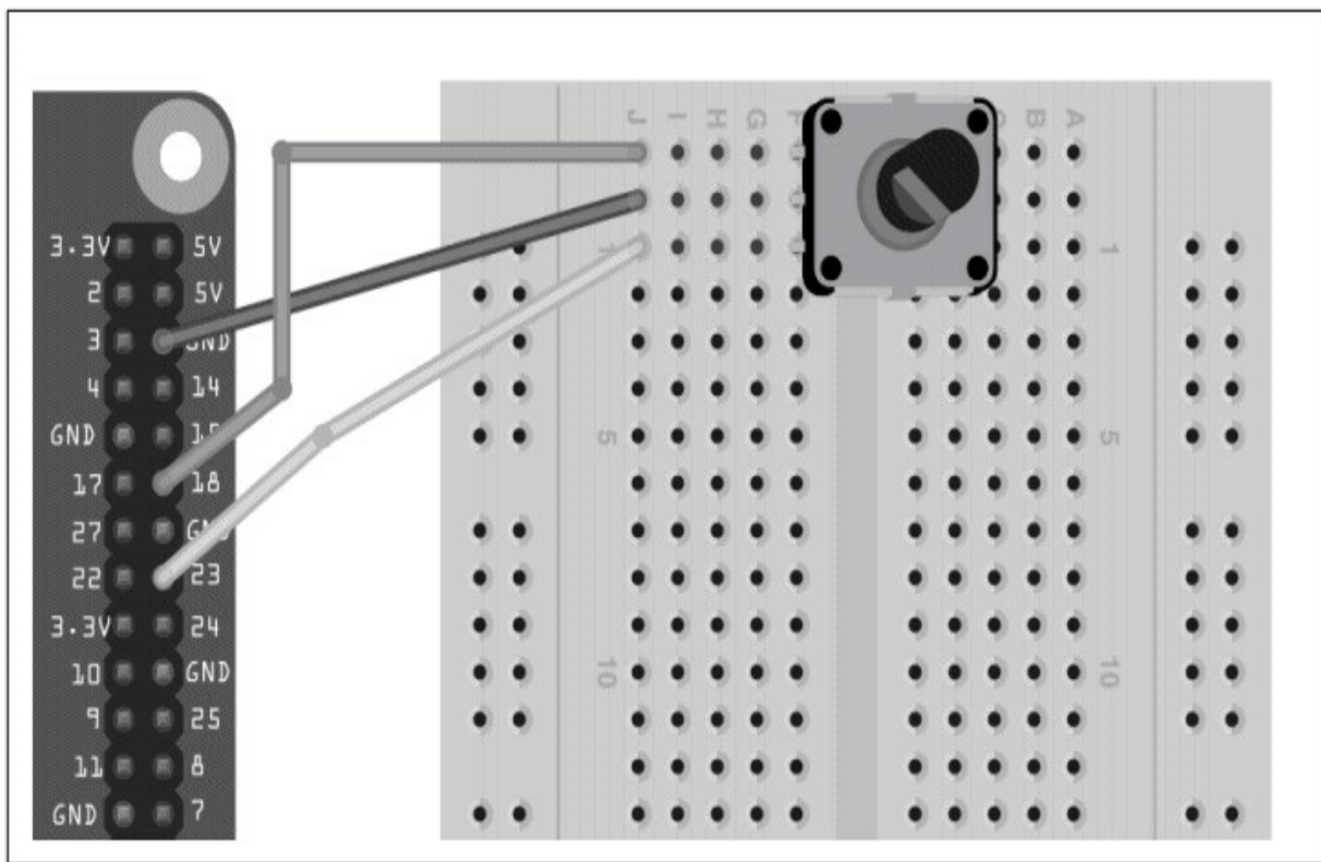
图12-10 连接旋转编码器
