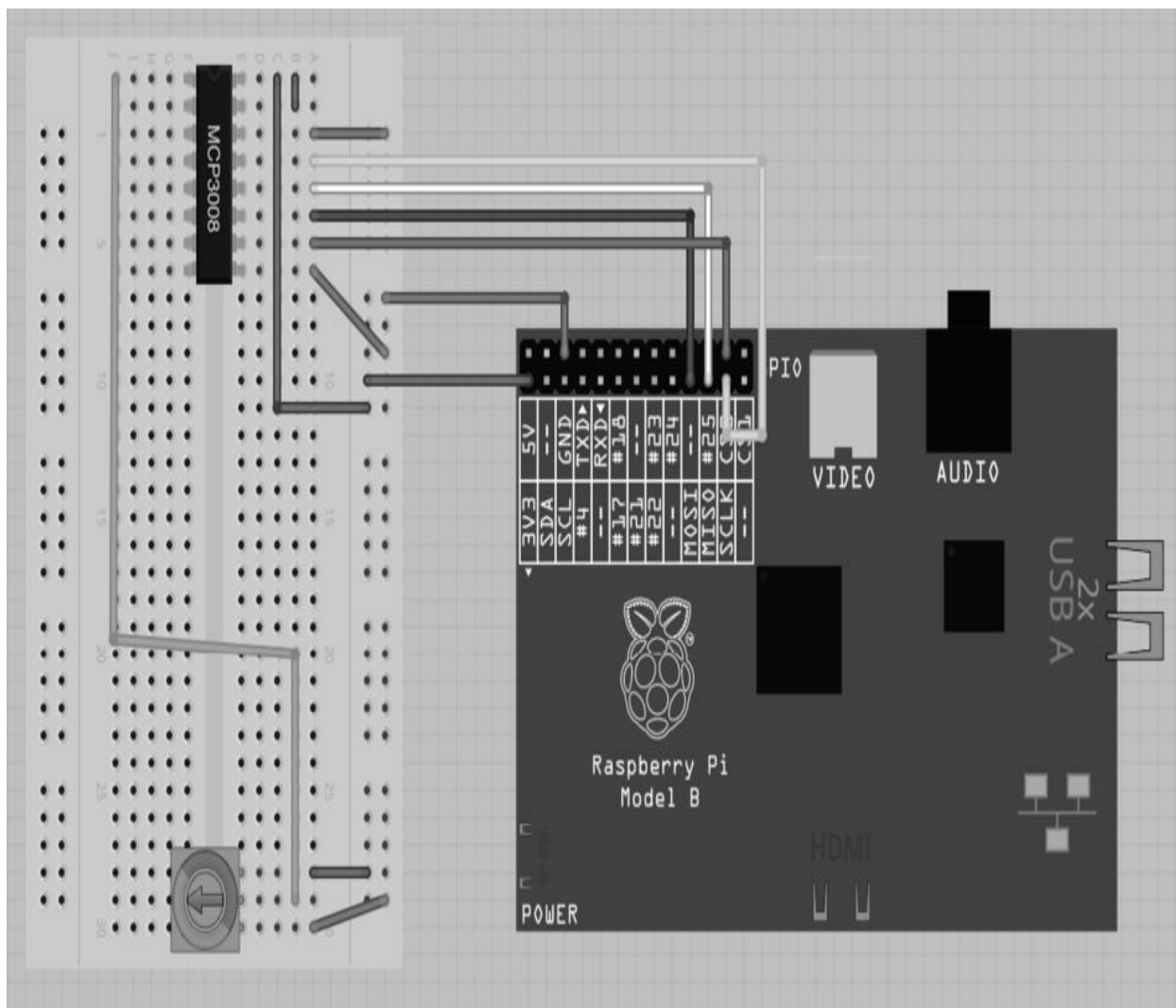
图13-11 在树莓派上面使用MCP3008 ADC IC
