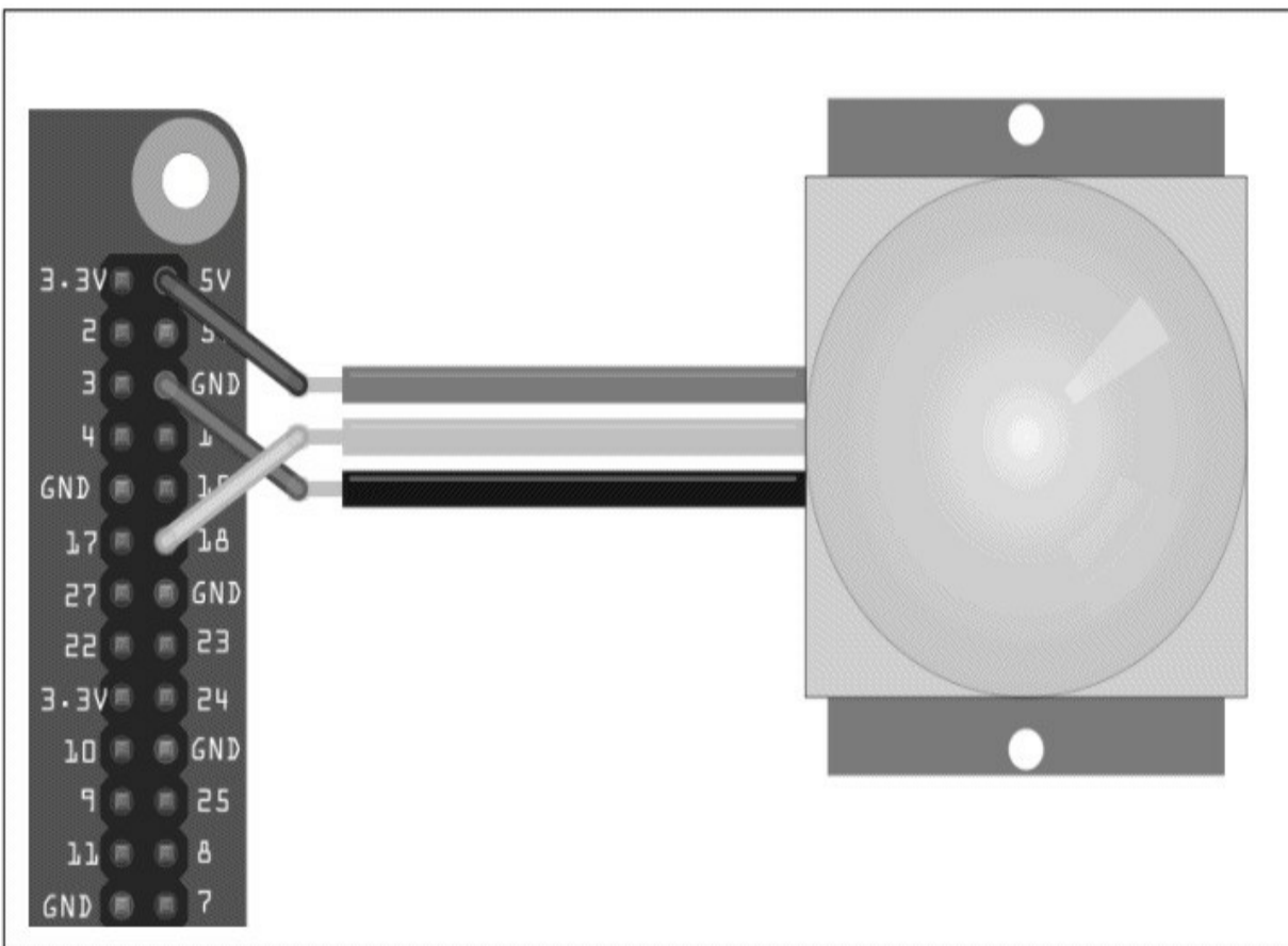
图12-14 连接PIR运动检测模块
