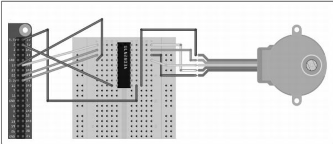
图11-12 使用ULN2803控制单极步进电机
