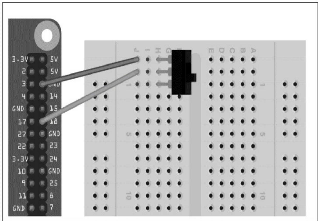
图12-5 将滑动开关连接到树莓派
