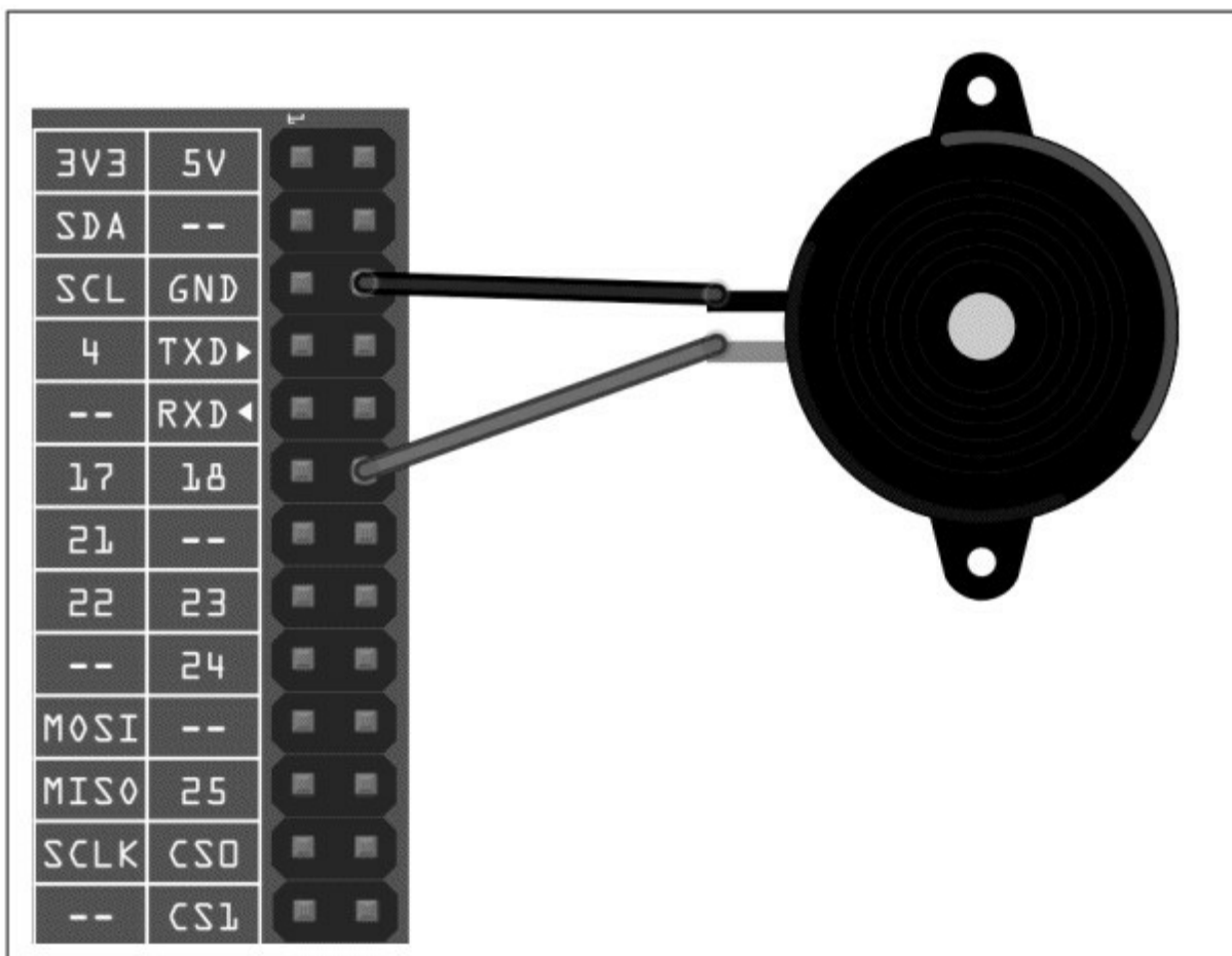
图10-3 为树莓派连接压电蜂鸣器
