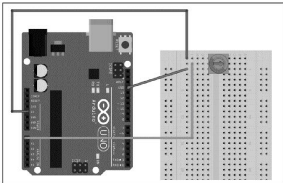
图16-10 Arduino与调谐电位器的布线图
