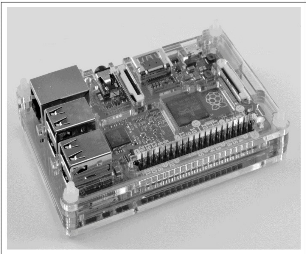
图1-2 安装在PiBow Coupé中的树莓派
