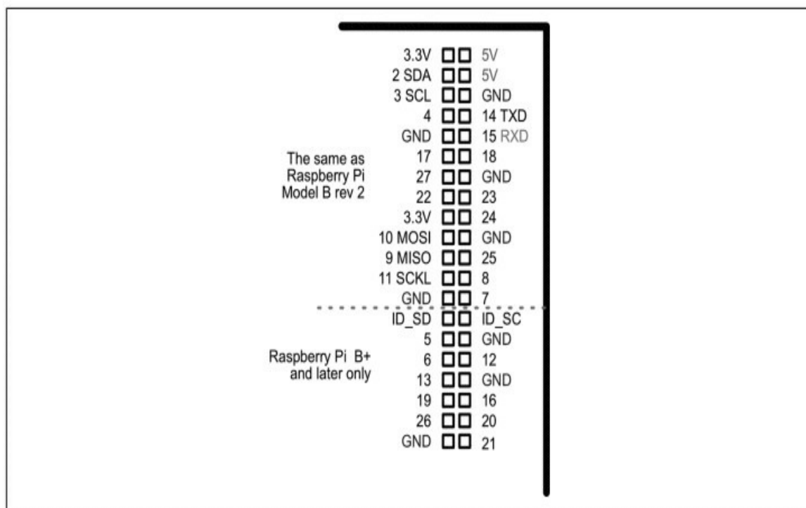
图9-2 GPIO引脚（40个引脚）
