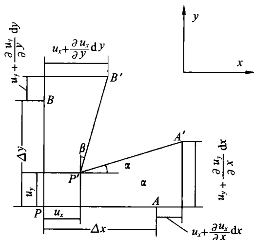
图 2.16 固体的形变
