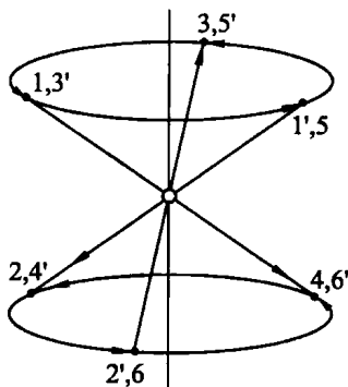
图 1.25 \bar{3} 的对称性
