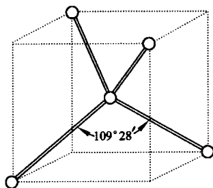
图 2.1 金刚石结构中的正四面体
