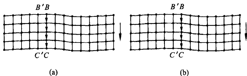
图 4.8 螺位错的滑移
