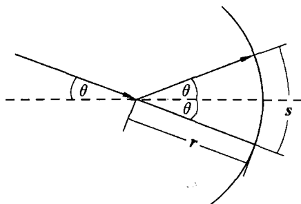
图 1.34 粉末衍射
