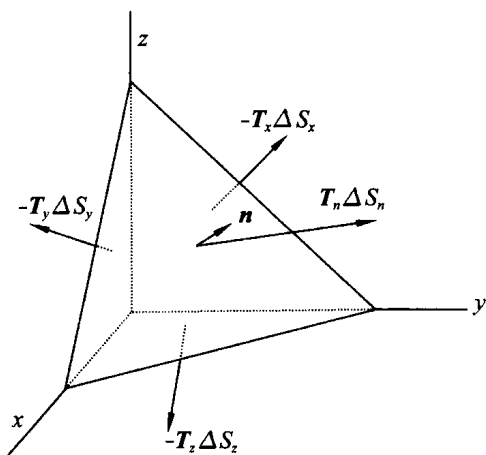
图 2.15 四面体体积元受到的应力
