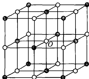
图 2.12 NaCl 结构的埃夫琴晶胞
