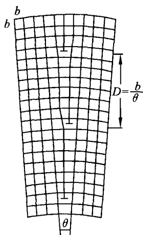
图 4.4 小角晶界的刃位错
