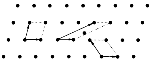
图 1.12 原胞选取的示意图
