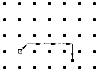
图 4.1 弗仑克尔缺陷
