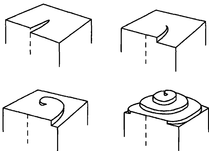
图 4.10 有螺位错的晶体的生长
