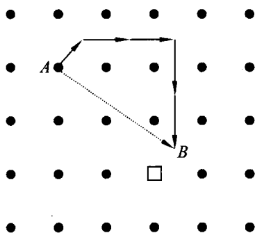
图 4.13 填隙原子的扩散
