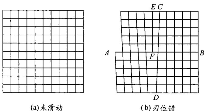
图 4.3 刃位错的形成
