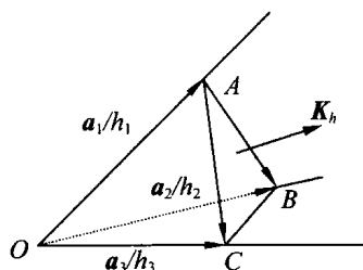
图 1.22 离原点最近的晶面
