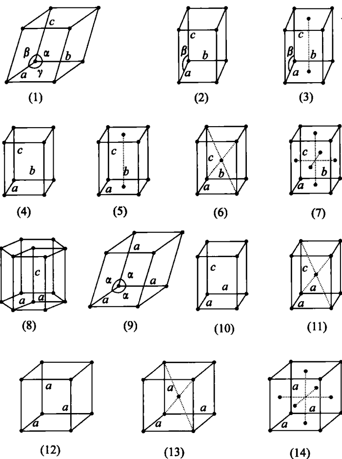
图 1.28 14 种布喇菲晶胞
