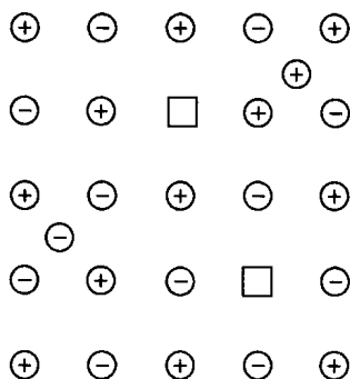
图 4.14 离子晶体中的缺陷
