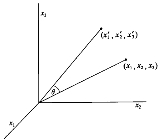
图 1.23 直角坐标的转动
