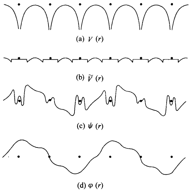
图 5.10 赝势 赝波函数
