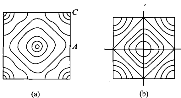
图 5.12 二维等能曲线 (a)近自由电子 (b)紧束缚电子
