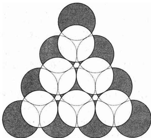
图 1.7 密堆积
