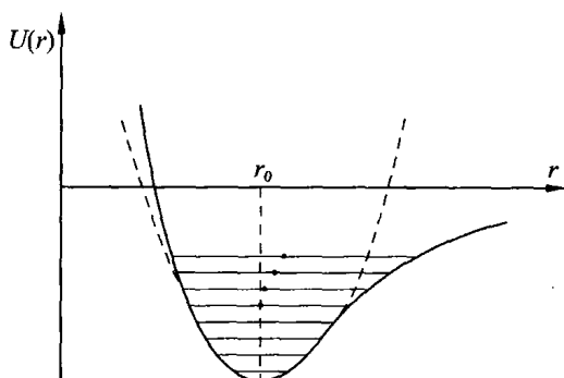
图 3.17 两原子间互作用势能曲线
