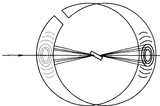
图 1.33 粉末衍射实验
