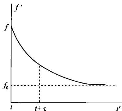
图 6.8 电子分布函数的恢复
