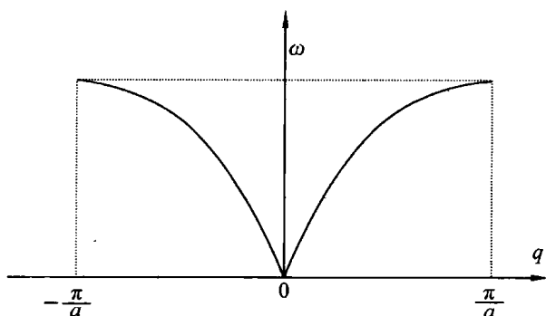
图 3.2 一维简单晶格的色散关系
