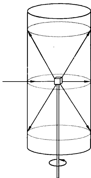
图 1.32 旋转单晶法示意图
