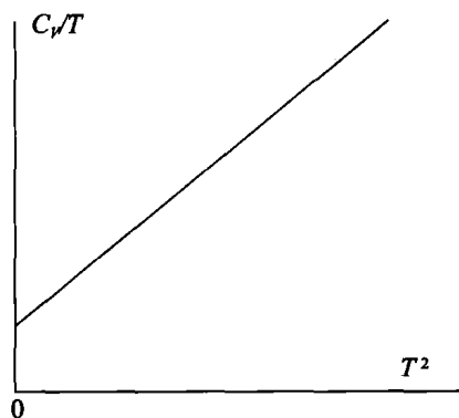
图 6.3 低温下 C_V/T \sim T^2 关系
