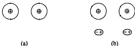
图 2.6 相邻氮原子的瞬时偶极矩
