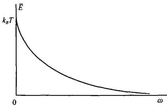
图 3.13 格波的振动能与频率的关系曲线
