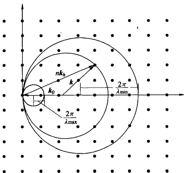
图 1.31 劳厄法的反射球
