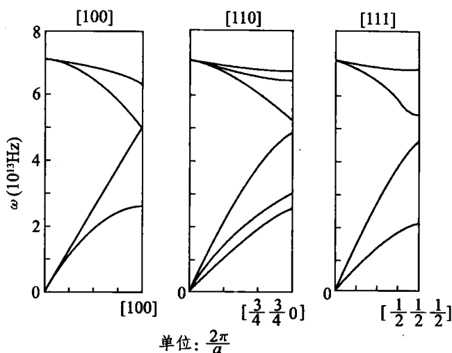
图 3.6 金刚石的振动谱
