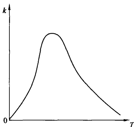
图 3.16 热导系数与温度的关系
