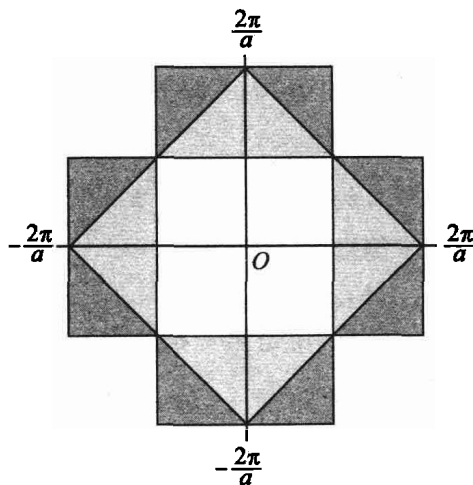
图 5.5 二维方格子布里渊区
