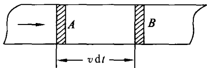
图 6.7 理想流体的漂移
