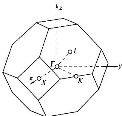
图 5.7 面心立方正格子第一布里渊区
