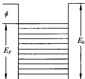
图 6.6 金属中电子的势阱
