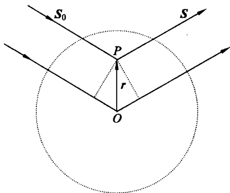
图 1.35 X 射线在原子中的散射
