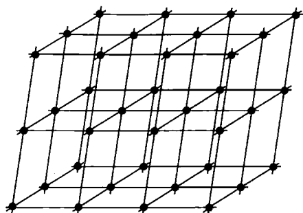
图 1.11 晶格
