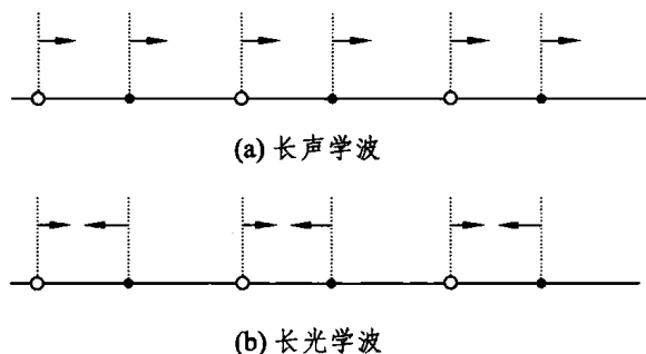
图 3.5 一维双原子链长波时原子的位移
