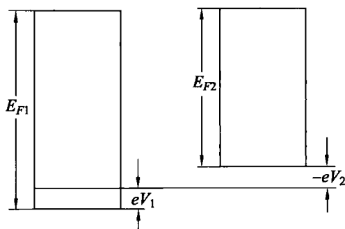
图 6.5 两金属接触平衡后价电子能级分布
