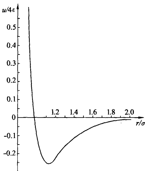
图 2.7 雷纳德—琼斯势
