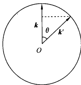
图 6.9 电子的弹性散射
