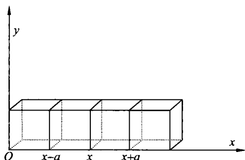
图 4.16 离子的扩散
