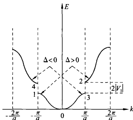
图 5.2 近自由电子的能带
