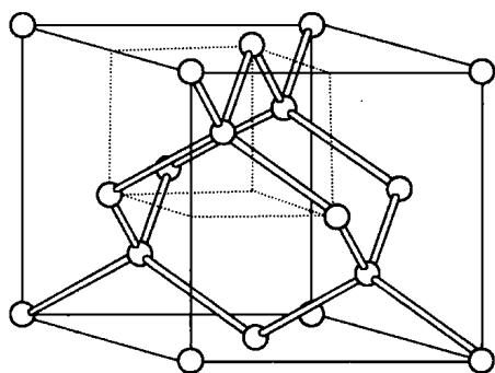
图 1.18 金刚石结构
