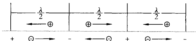
图 3.9 离子晶体的宏观极化
