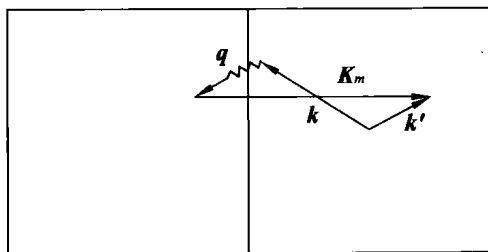
图 6.10 电子的倒逆过程
