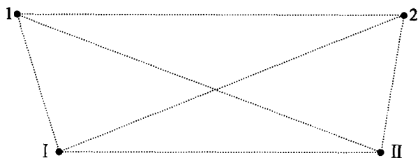
图 2.8 两氢原子的相互作用
