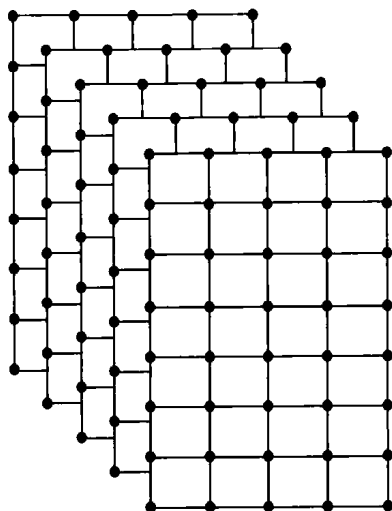
图 1.20 晶面族
