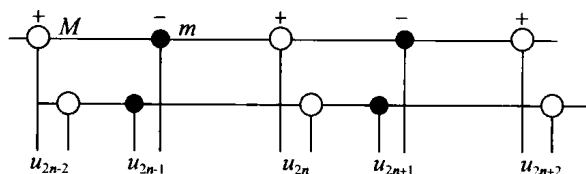
图 3.10 一维离子晶格的离子位移
