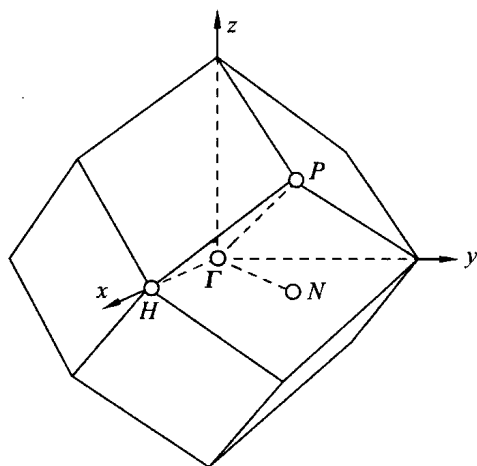
图 5.6 菱形十二面体
