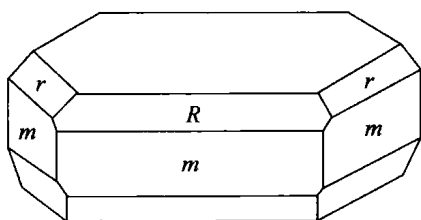
图 1.2 一种人造石英
