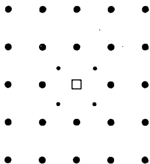
图 4.12 空位附近的间隙位置
