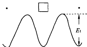
图 4.11 空位周围的势垒
