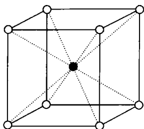
图 1.16 氯化铯结构
