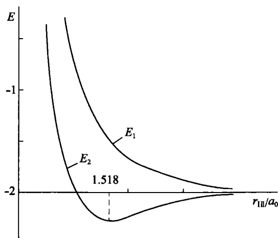
图 2.9 氢分子的能量与氢原子间距的关系
