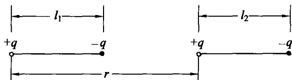
图 2.4 一对平行偶极子的相互作用
