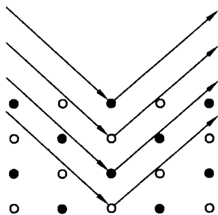
图 1.36 复式格子的布拉格反射
