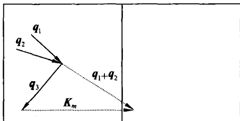
图 3.15 声子的倒逆过程
