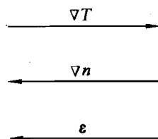
图 6.13 \nabla T 、 \nabla n 和 \epsilon 的方向
