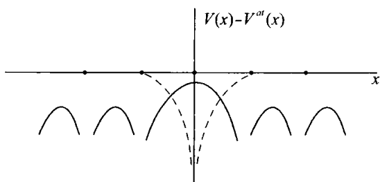
图 5.8 移去一原子的一维势场
