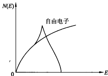
图 5.14 自由电子和近自由电子的能态密度
