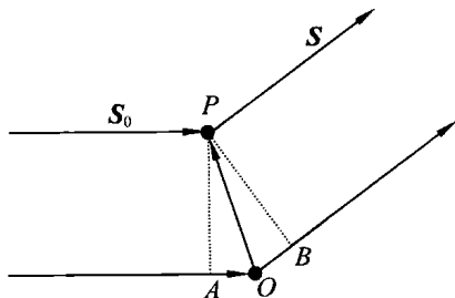
图 1.21 X 射线衍射
