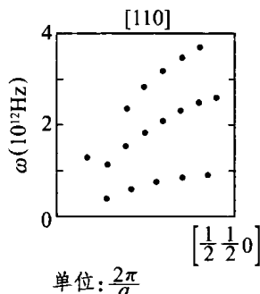
图 3.8 钠金属 90K 时[110]方向的振动谱
