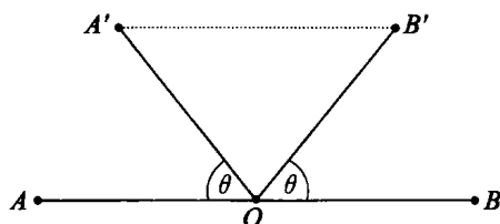
图 1.24 一晶面上的晶列
