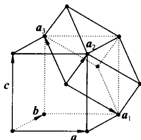
图 1.14 体心立方
