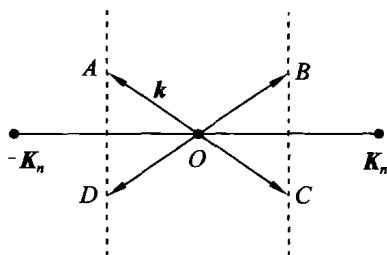
图 5.11 布里渊区界与波矢 \mathbf{k}
