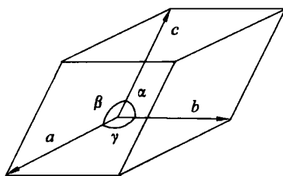
图 1.27 晶胞
