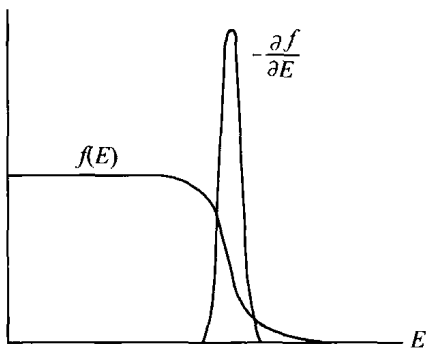
图 6.2 f(E) 与 \left(-\frac{\partial f}{\partial E}\right)
