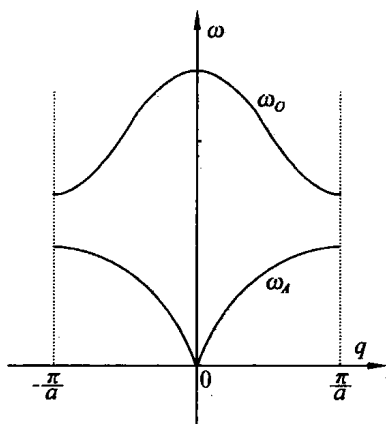
图 3.4 一维双原子晶格的频谱
