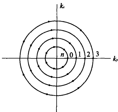
图 5.16 磁场中电子的量子态分布
