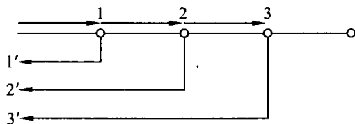
图 5.1 一维晶格的布拉格反射
