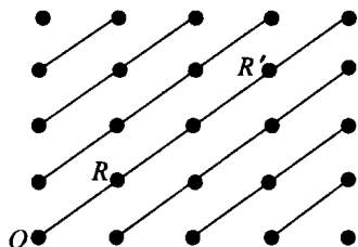
图 1.19 晶列
