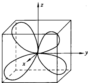
图 2.11 碳原子的杂化轨道
