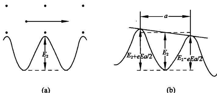
图 4.15 有外电场前后势垒的变化
