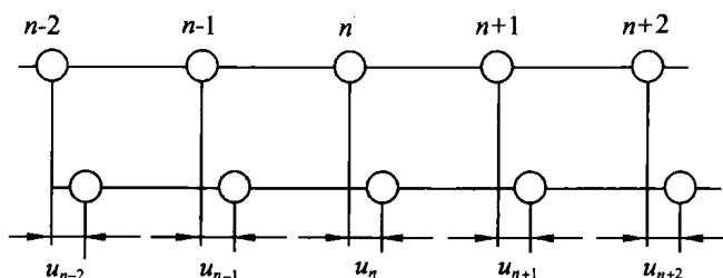
图 3.1 一维简单晶格的振动
