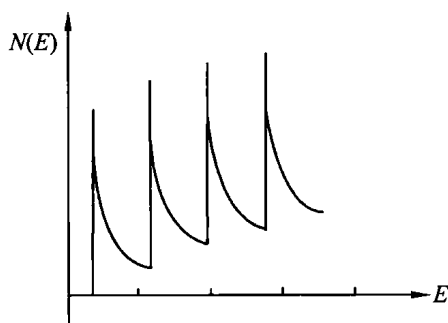
图 5.17 磁场中电子的能态密度
