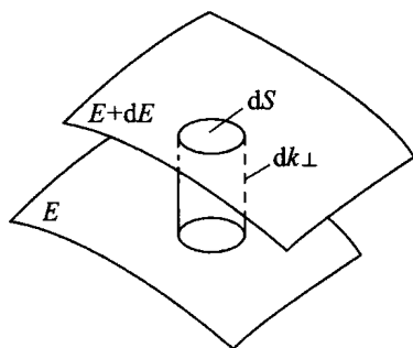
图 5.13 波矢空间内两等能面间体积元
