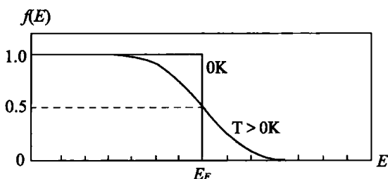
图 6.1 不同温度下的费密分布
