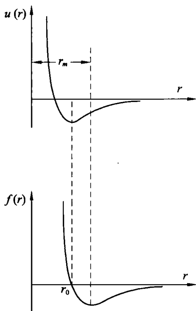
图 2.2 原子间的相互作用
