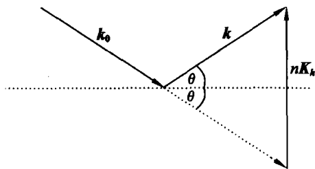
图 1.29 晶格的布拉格反射
