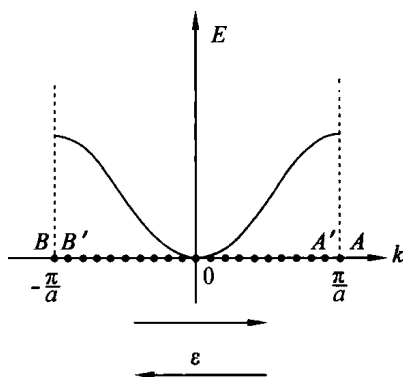
图 5.18 满带
