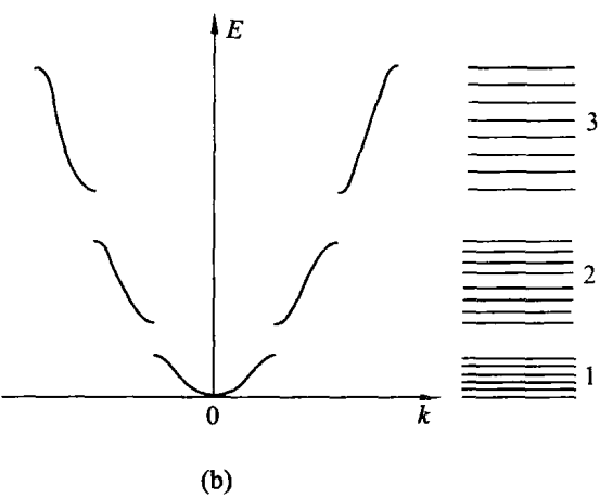
图 5.3 能带 (a)周期性表示和简约布里渊区表示; (b)抛物线型表示
