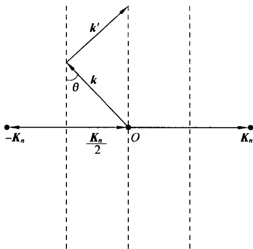
图 5.4 电子的布拉格反射
