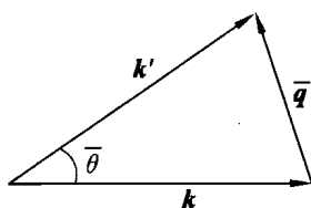
图 6.12 电子正常散射
