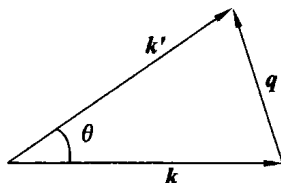
图 3.7 光子散射
