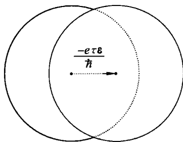
图 6.11 在外电场中费密球的平移
