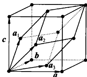
图 1.15 面心立方
