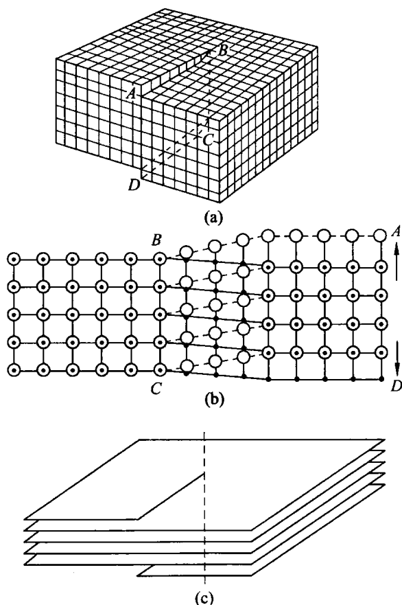
图 4.5 螺位错
