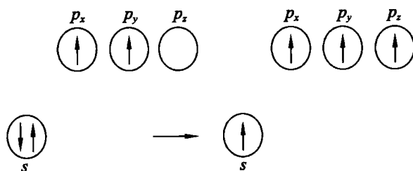
图 2.10 碳原子的基态和激发态
