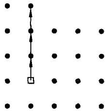
图 4.2 肖特基缺陷
