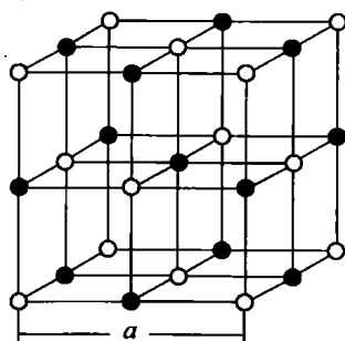
图 1.17 氯化钠结构
