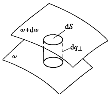
图 3.11 波矢空间内一支格波的等频面
