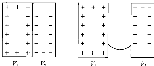
图 6.4 金属接触电势差
