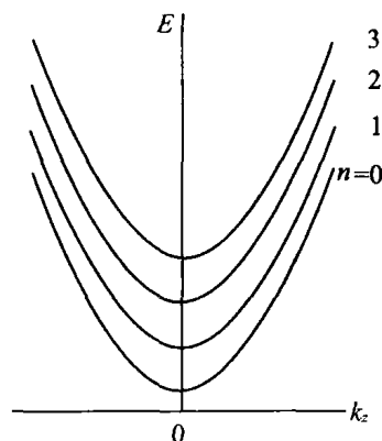
图 5.15 自由电子在磁场中的能带
