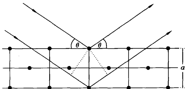
图 1.30 体心立方晶体 (001) 面的一级衍射
