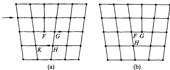
图 4.7 刃位错附近原子的受力情况
