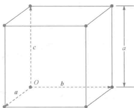
图 1.10 立方晶系的晶胞
