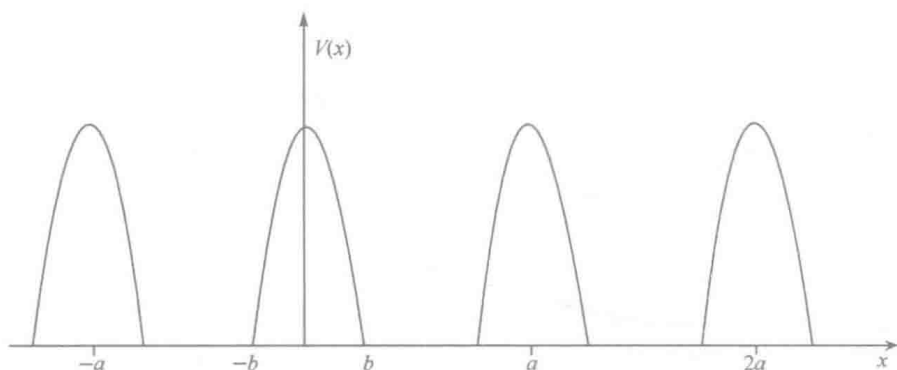
图 1.62 一维周期势场
