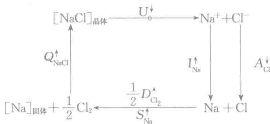
图 1.28 玻恩-哈伯循环
